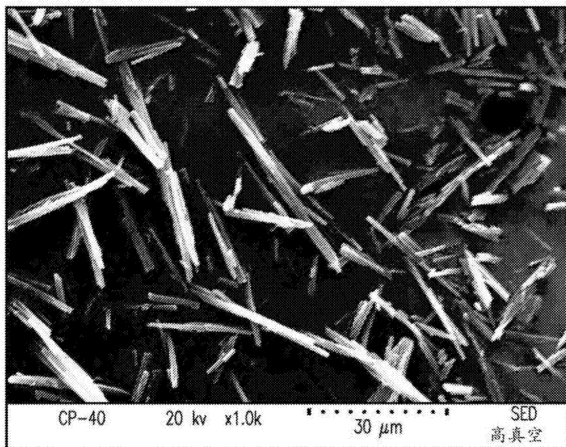
化合物(I-S) HCl盐A型的晶癖
