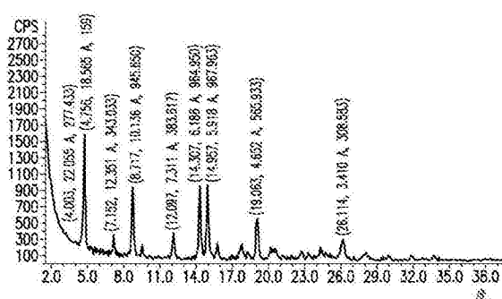
化合物(1-S)的粉末XRPD图案
