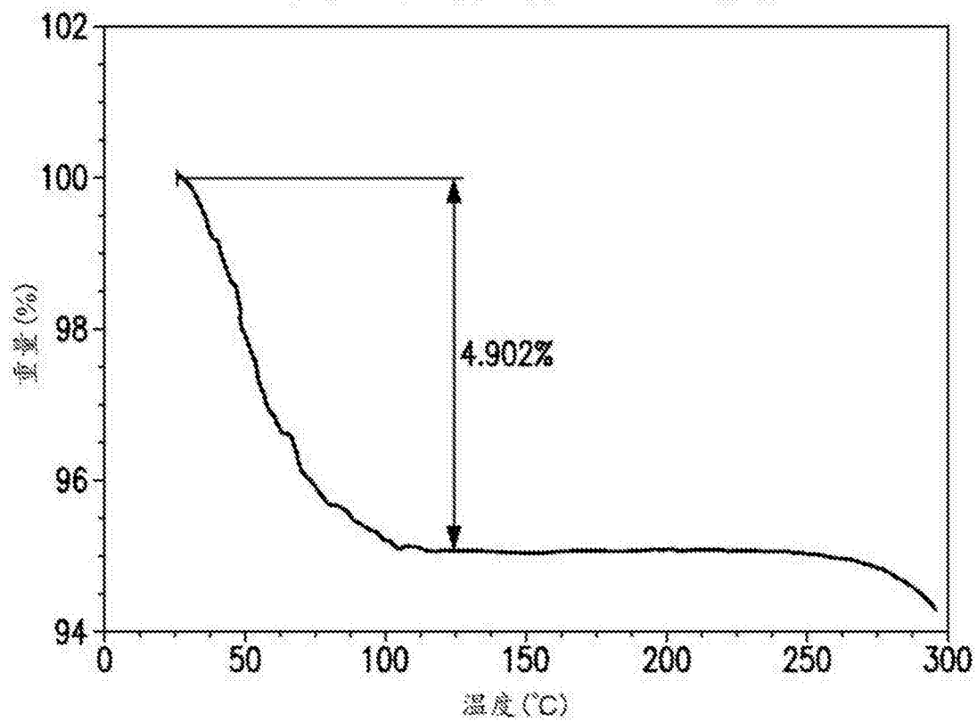
外消旋化合物(I)的水合物的TGA图谱图
