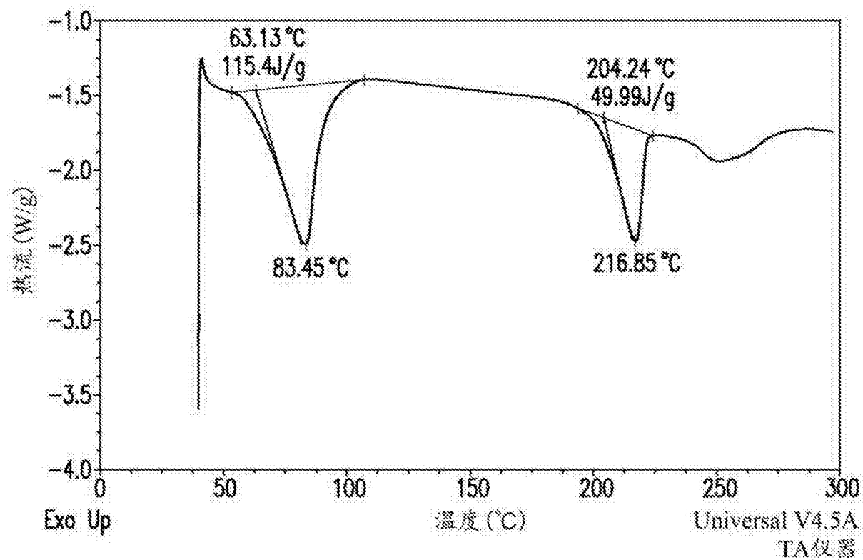
化合物(I-S) HCl盐F型的DSC温谱图
