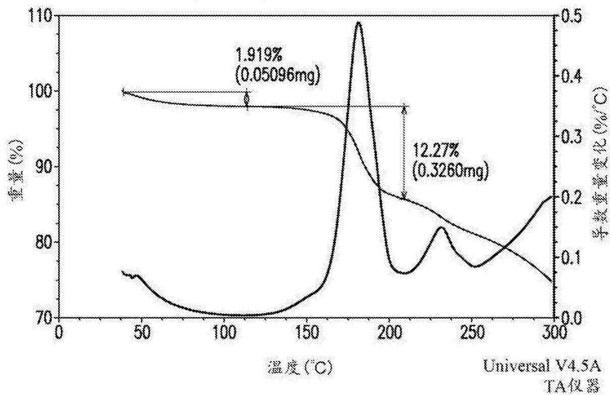
化合物(I-S) HCl盐G型的TGA图谱图
