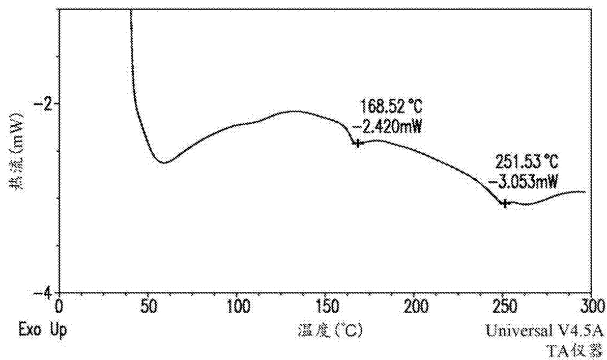
化合物(I-S) HCl盐D型的DSC温谱图
