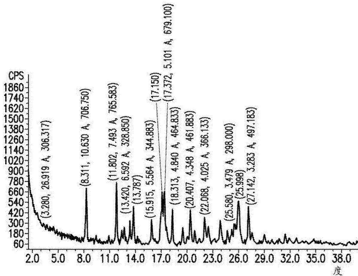
化合物(I-S)的水合物的XRPD图案
