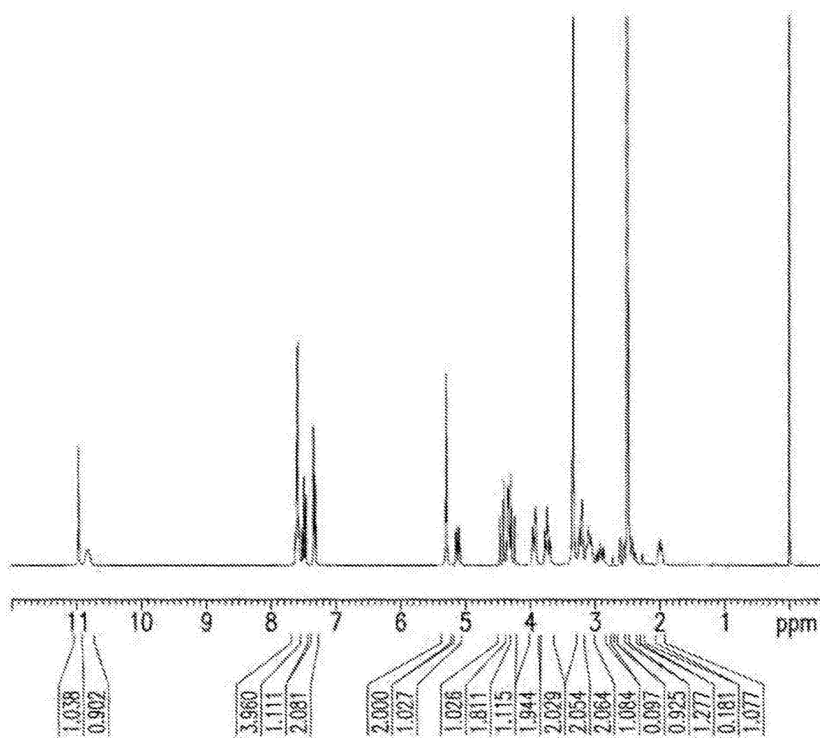
化合物(I-S) HCl盐E型的 1 H-NMR谱
