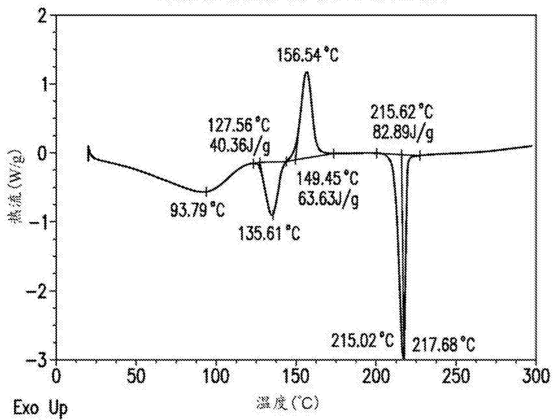
外消旋化合物(I)的水合物的DSC温谱图
