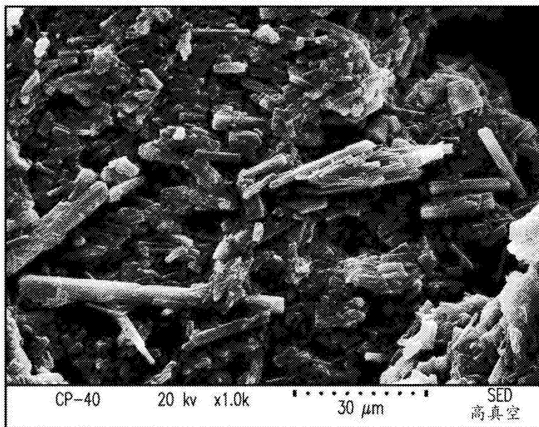
化合物(I-S) HCl盐C型的晶癖
