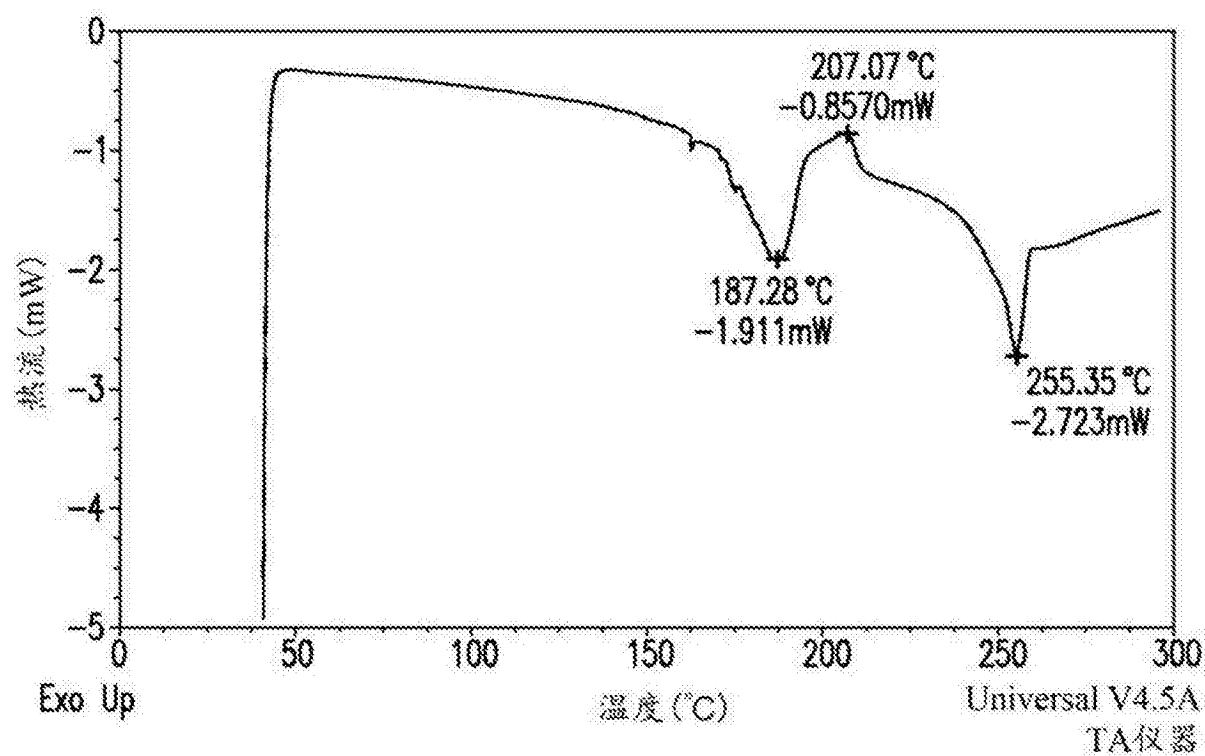
化合物(I-S) HCl盐H型的DSC温谱图
