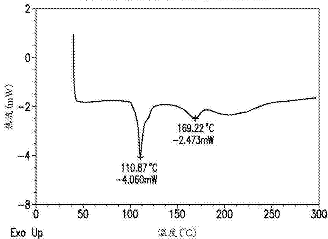
化合物(I-S)的半D-酒石酸盐的DSC温谱图
