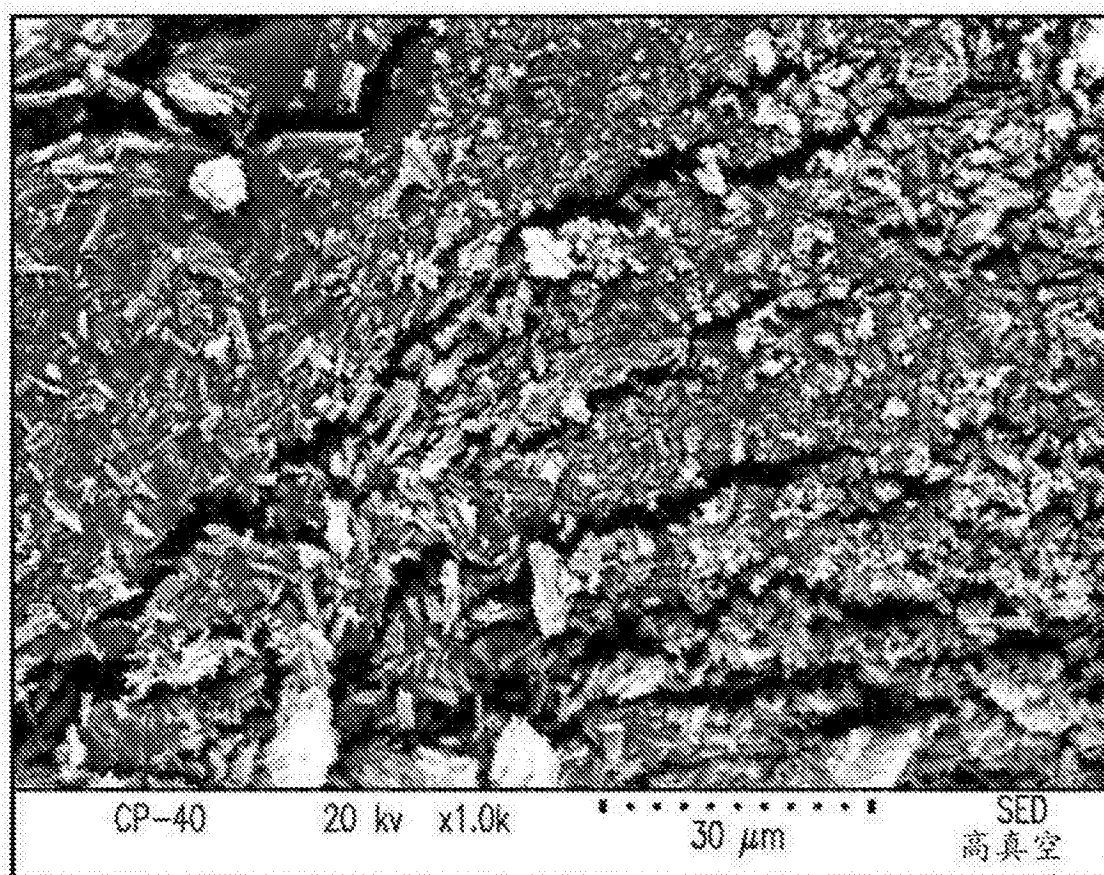
化合物(I-S) HCl盐D型的晶癖
