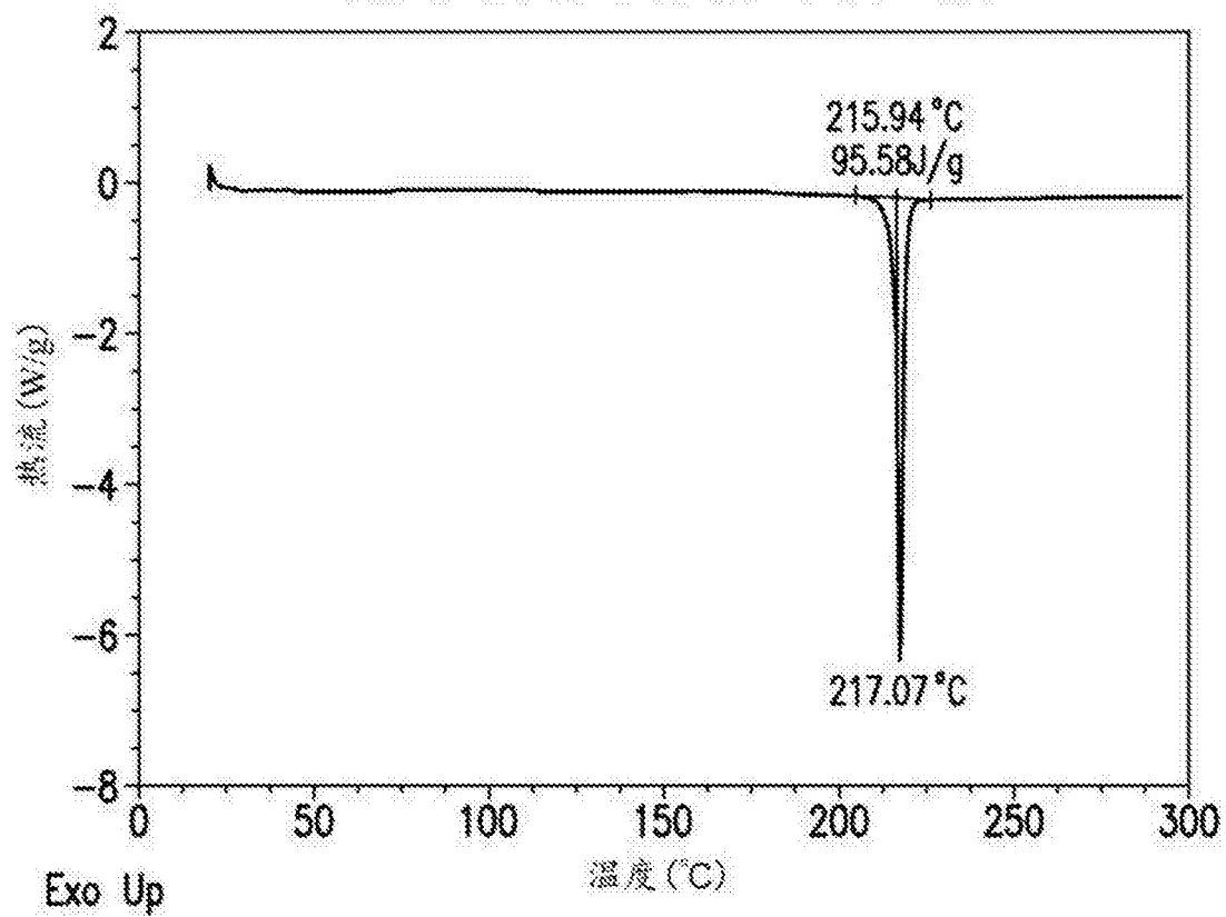
外消旋化合物(I)的无水合物的DSC温谱图
