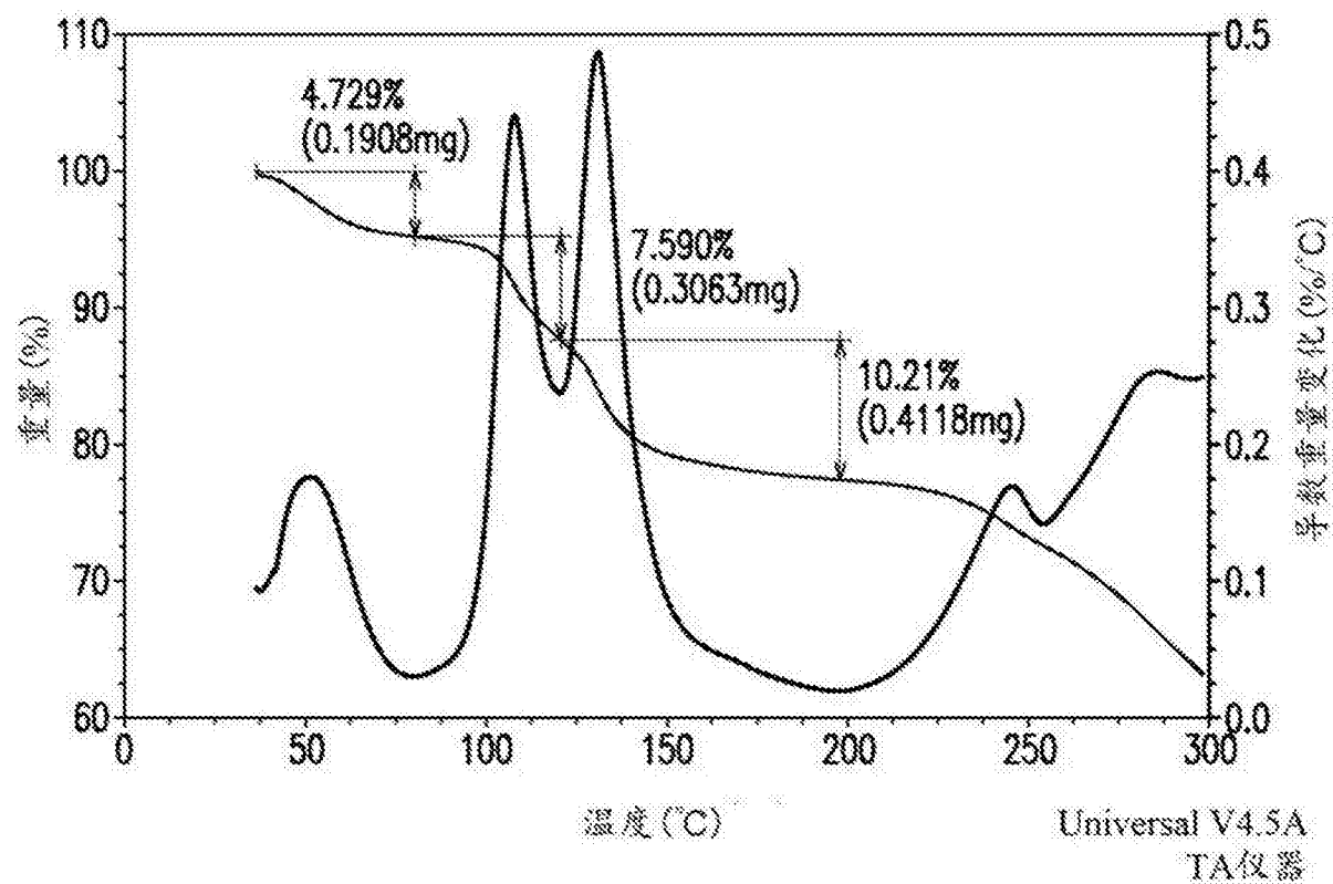
化合物(I-S) HCl盐J型的TGA温谱图
