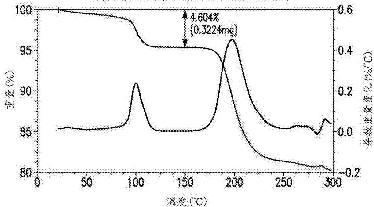
化合物(I-S)的半D-酒石酸盐的TGA温谱图
