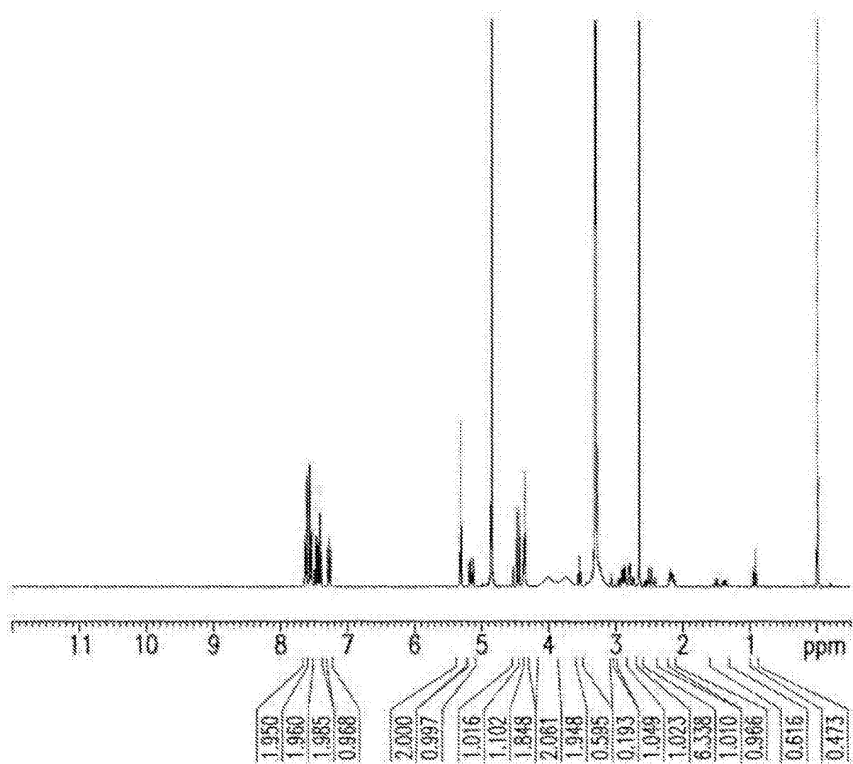
化合物(I-S) HCl盐C型的 1 H-NMR谱
