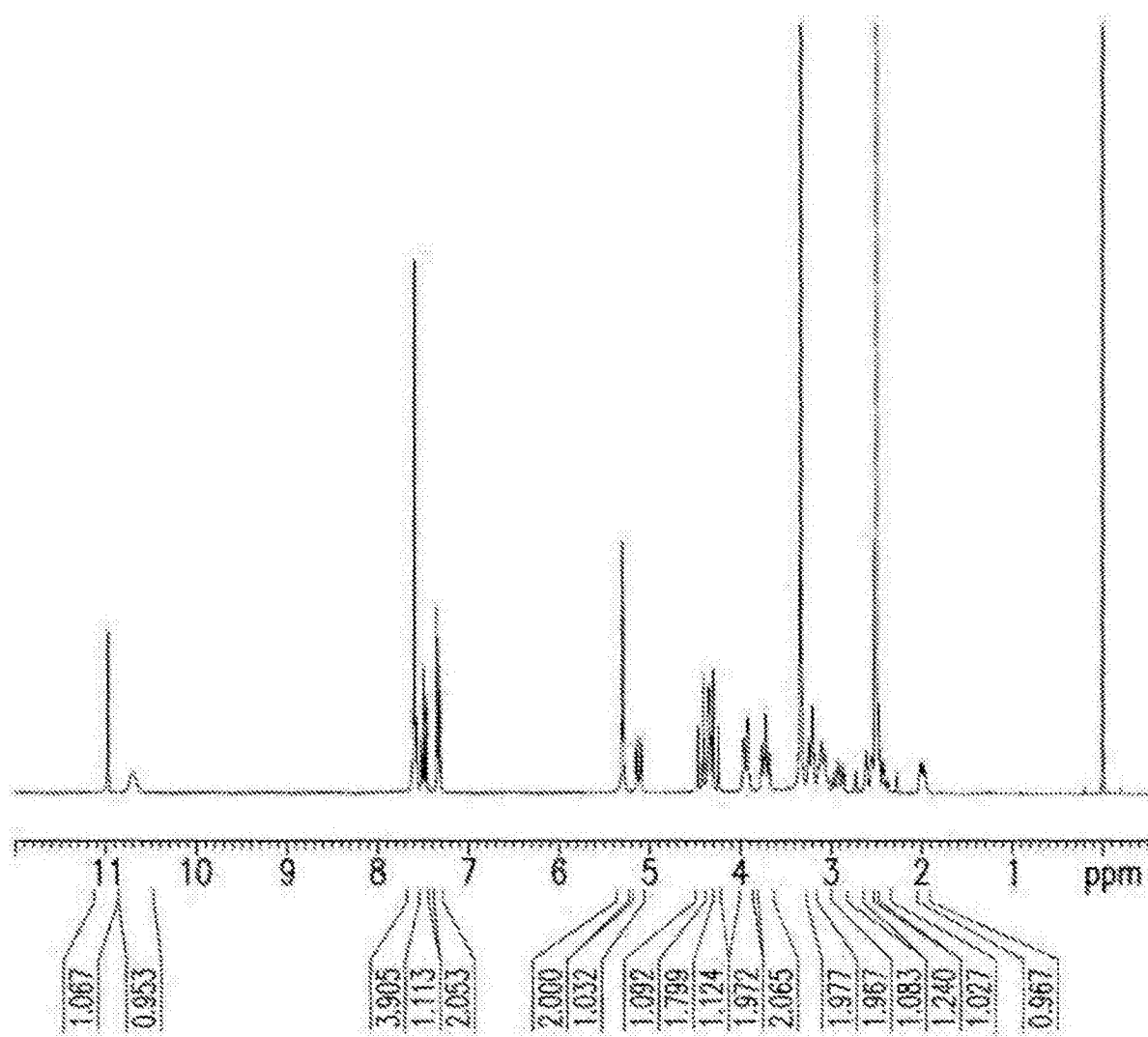
化合物(I-S) HCl盐D型的 1 H-NMR谱
