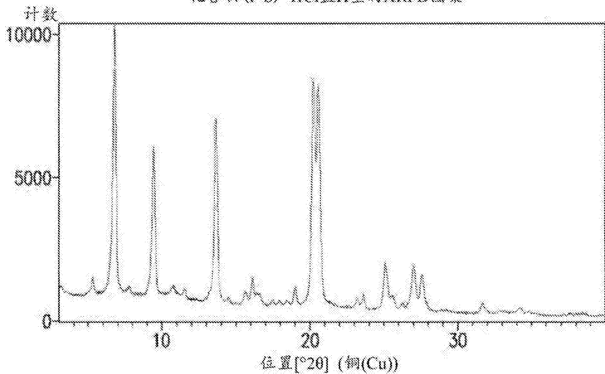
化合物(I-S) HCl盐H型的XRPD图案
