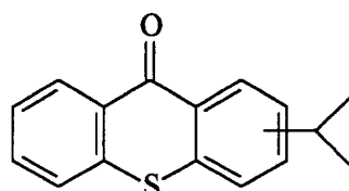
Isopropylthioxanthone ITX
