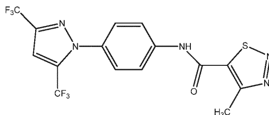
YM-58483
