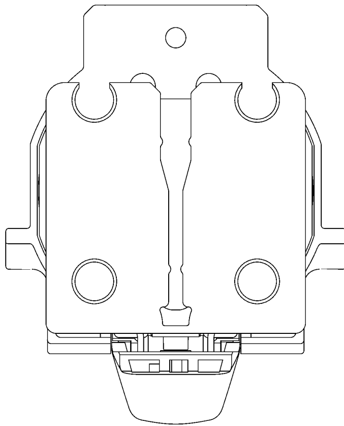
【後視圖】
