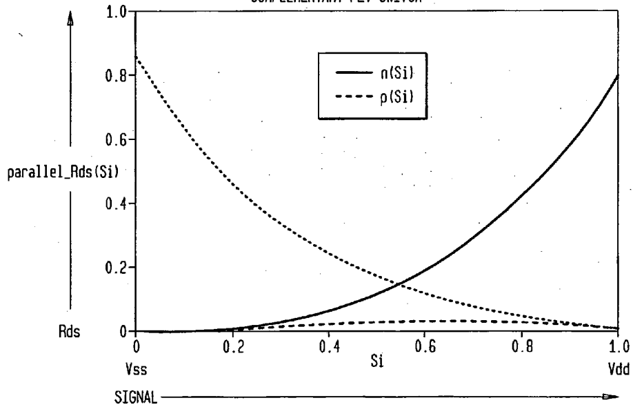
FIG. 241 COMPLEMENTARY FET SWITCH
