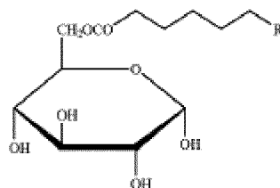
Glucosefetttsäureester
