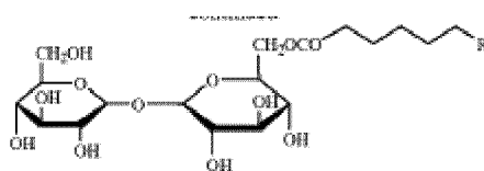
Trehalosefetttsäureester
