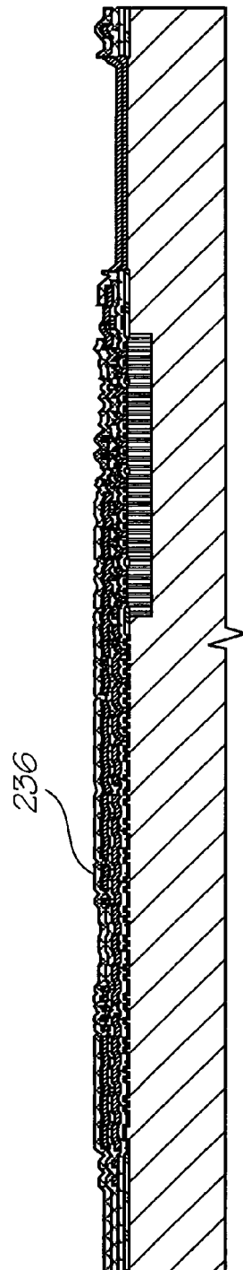
Deposit ILD 3, etch vias
