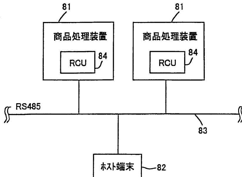
従来の管理システムの構成図
