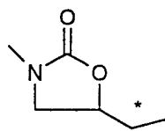
(B) (Enantiomer)
