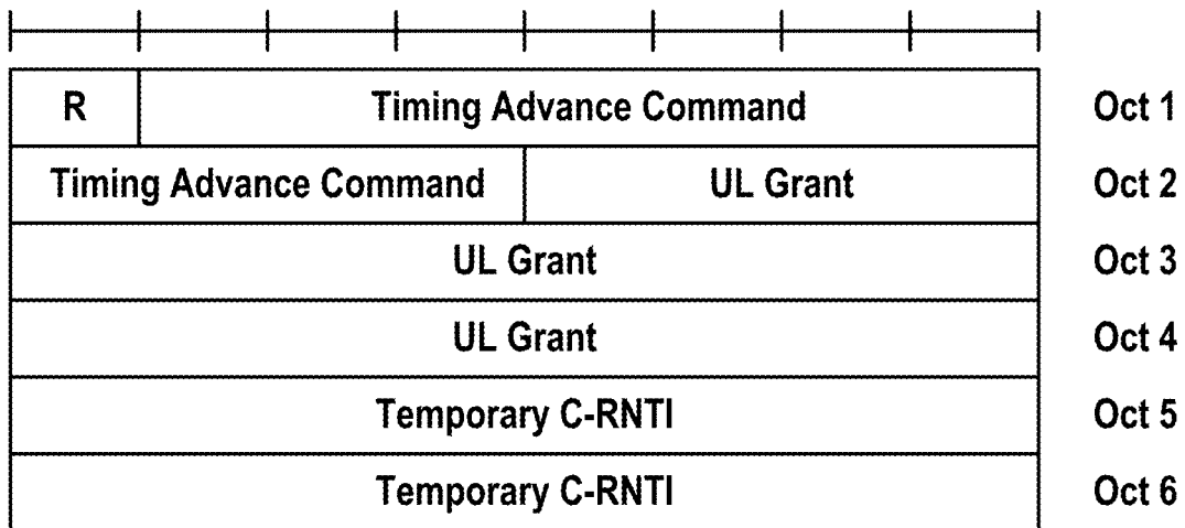
MAC RAR FIG. 18A
