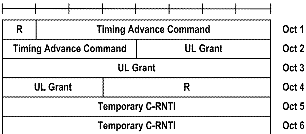
MAC RAR for NB-IoT UEs FIG. 18C
