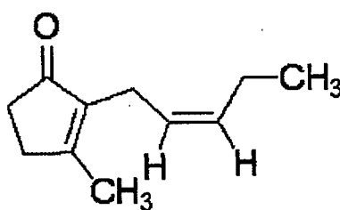
Jasmone
