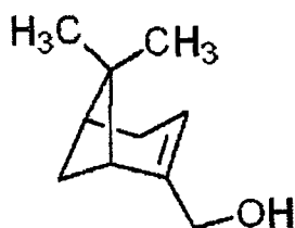
Myrtenol
