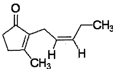
Jasmone
