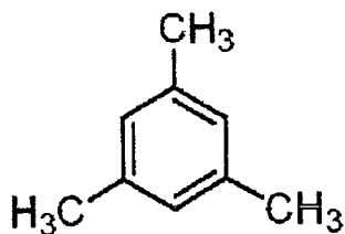
1,3,5-Trimethylbenzene
