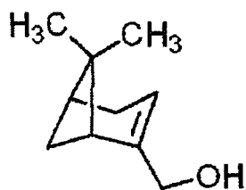
Myrtenol
