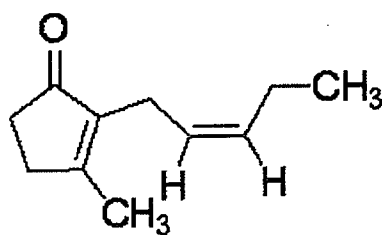
Jasmone
