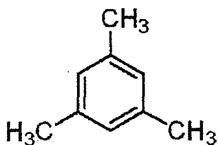
1,3,5-Trimethylbenzene
