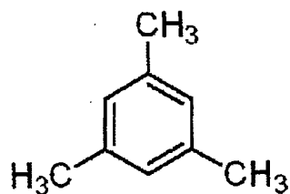
1,3,5-Trimethylbenzene
