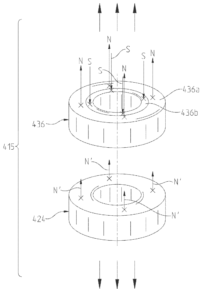
FIG. 12B
