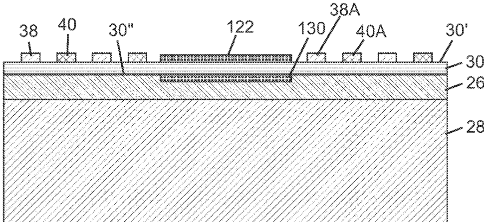
FIG. 24B
