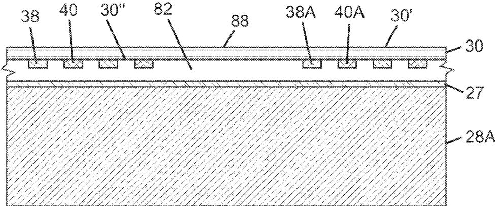
FIG. 19B
