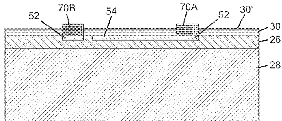
FIG. 14D
