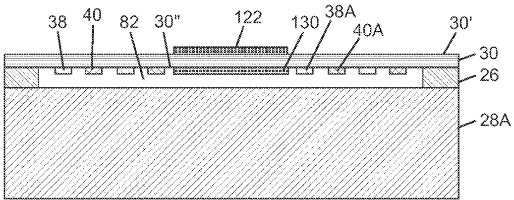
FIG. 25A
