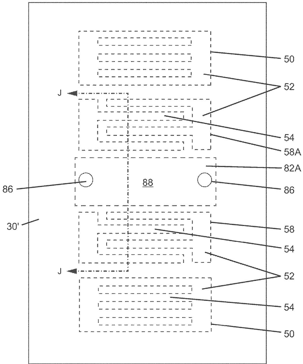
84 ↑ FIG. 20A
