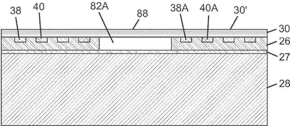
FIG. 20B
