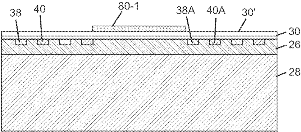
FIG. 17B
