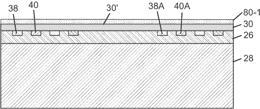
FIG. 16B
