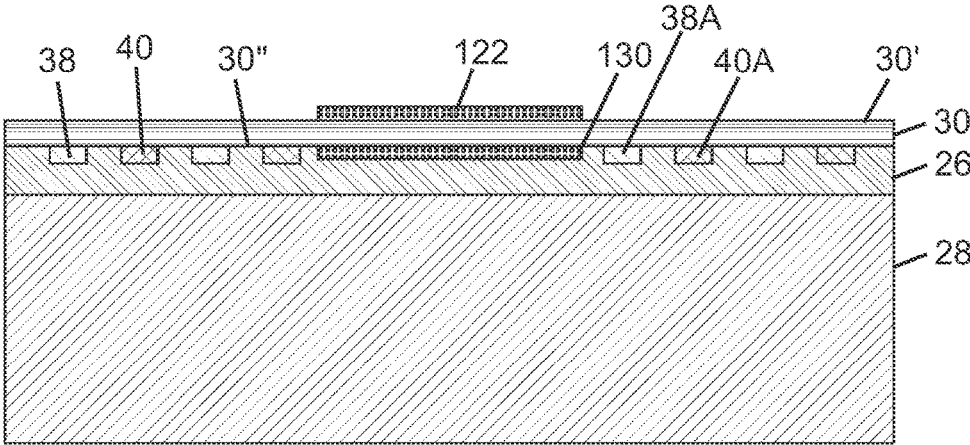
FIG. 24A
