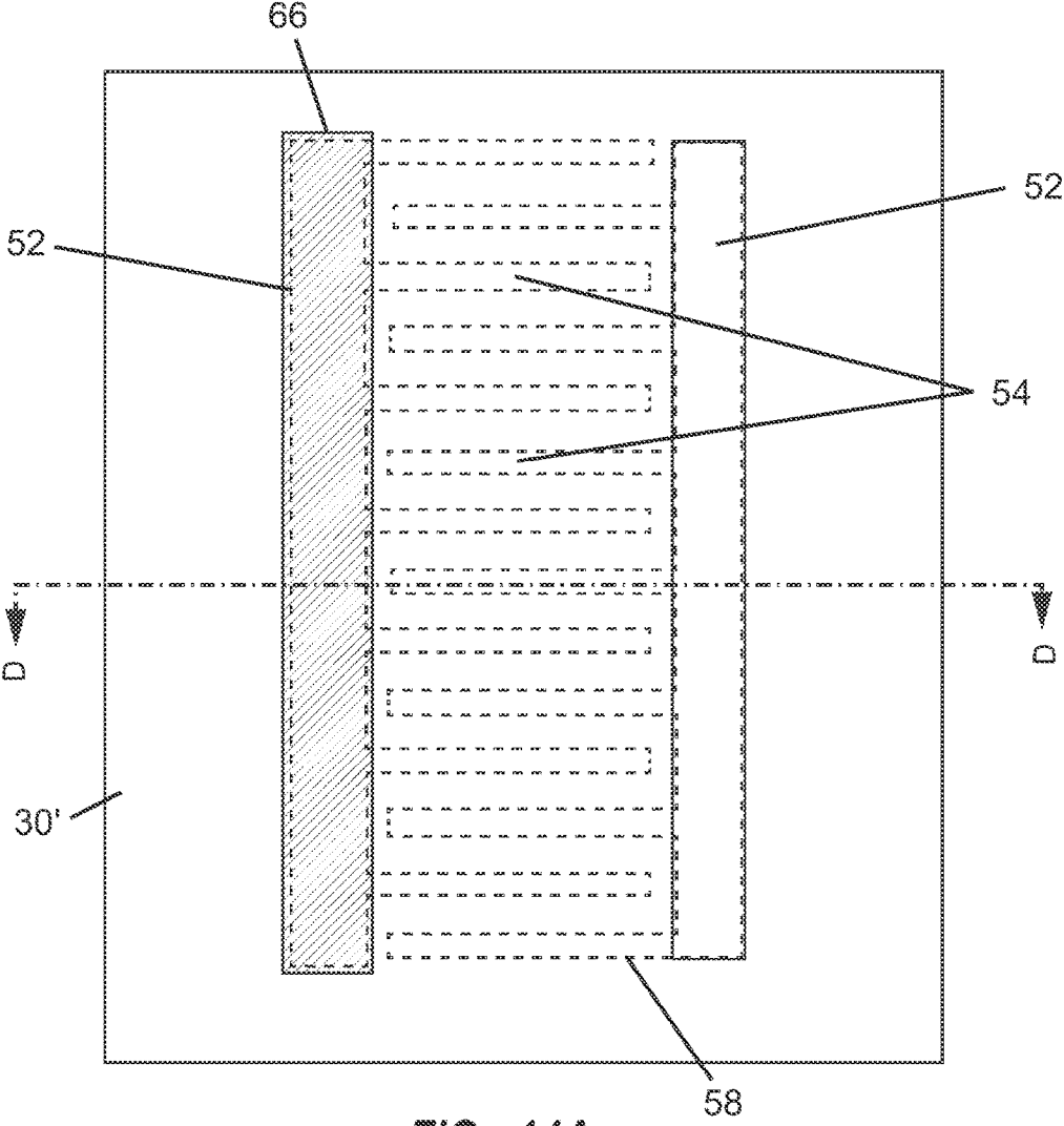
FIG. 14A
