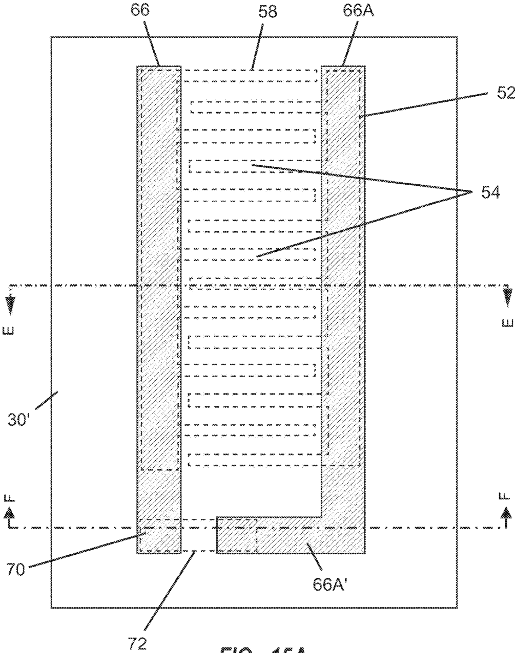
FIG. 15A
