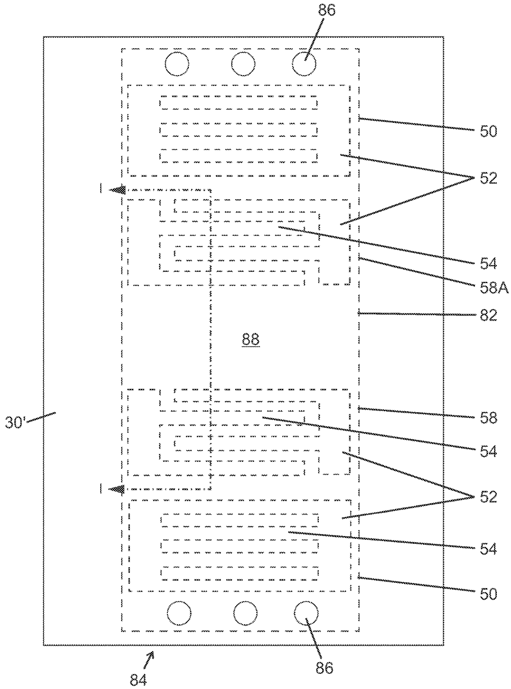
FIG. 19A
