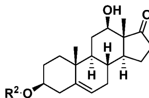
Formula I-15;
