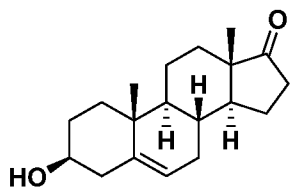
DHEA
