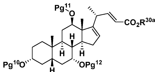
Formula III-4a.
