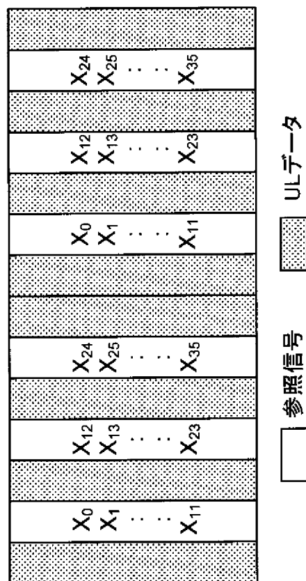
UL Grant フリー送信用チャネル構成
