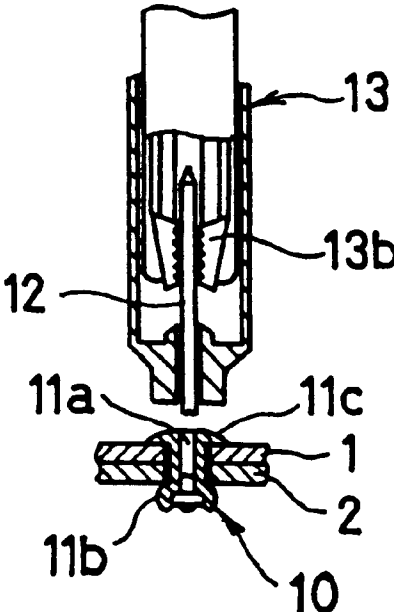
FIG. 95(d) (Prior Art)
