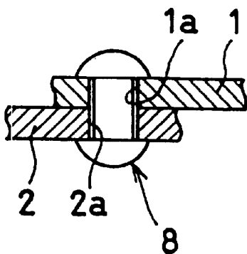
FIG. 94(d) (Prior Art)
