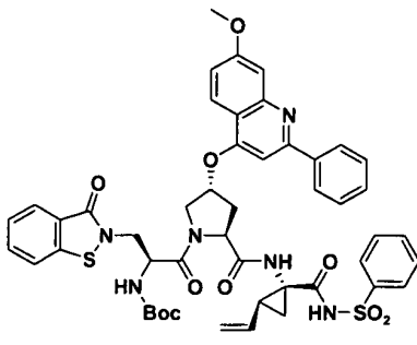
I-10
