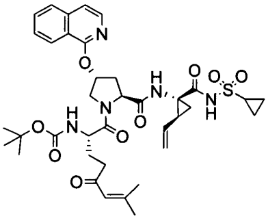
I-86
