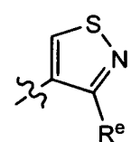
ccc
