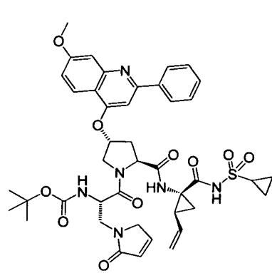
I-80
