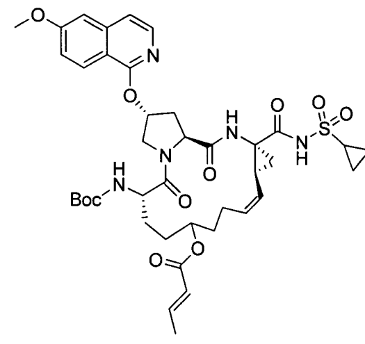
I-126
