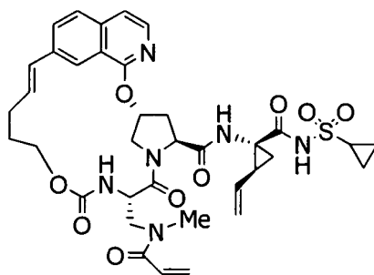
I-83
