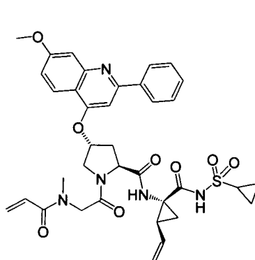
I-37
