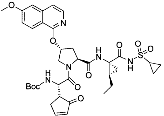
I-124
