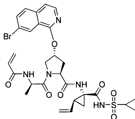
化合物 I-74
