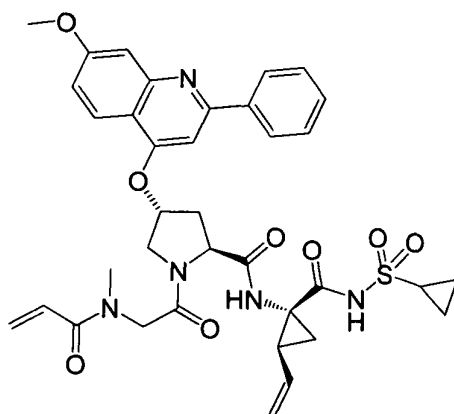
化合物 I-37
