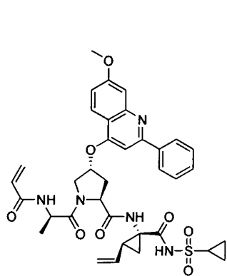
I-54
