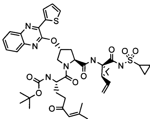
I-110
