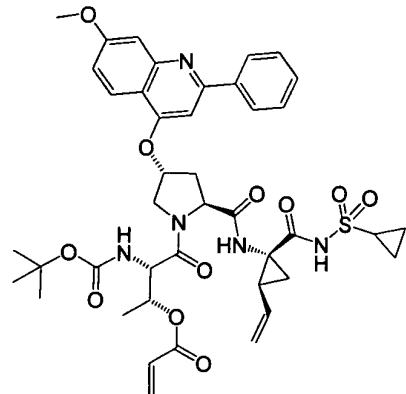
I-64
