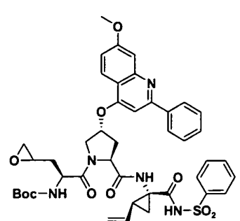
I-6
