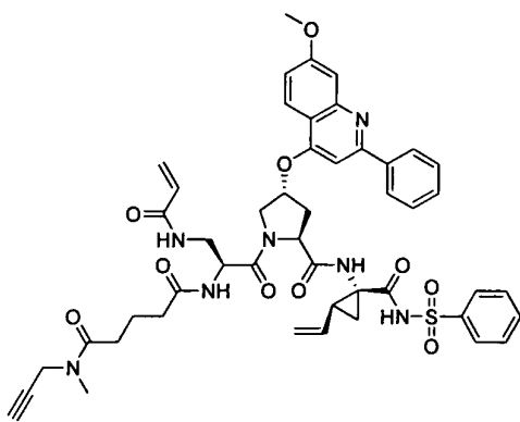
I-42
