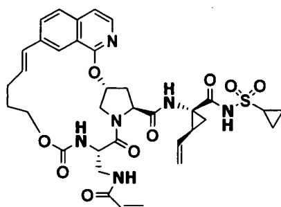
化合物 I-77
