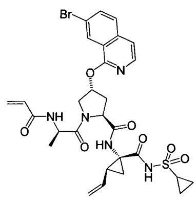
I-74
