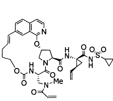
I-83
