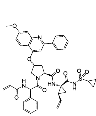
I-66
