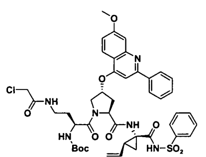
I-4
