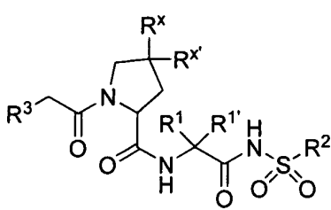
VIII-b
