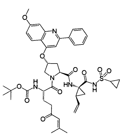
I-68
