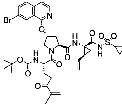
I-90
