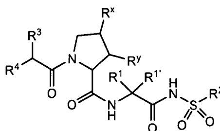
VI-b
