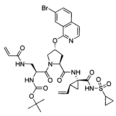
I-73
