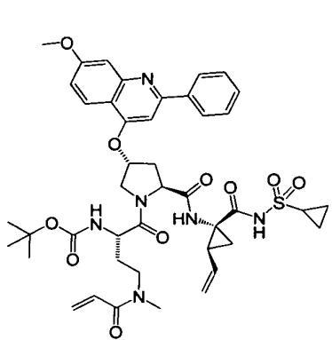
I-82
