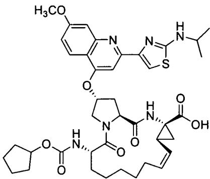
BILN 2061
