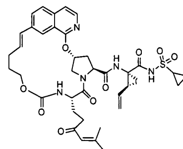
I-102
