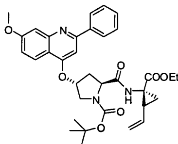
中間體1
