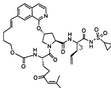
I-102
