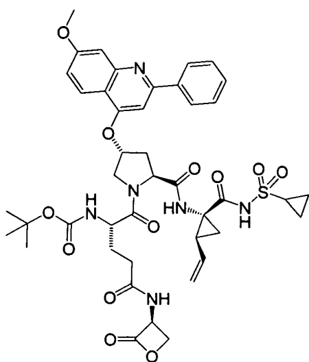
化合物 I-69
