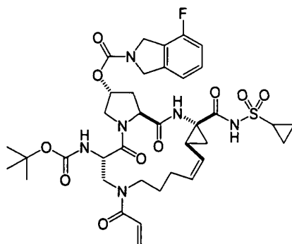
化合物 I-19
