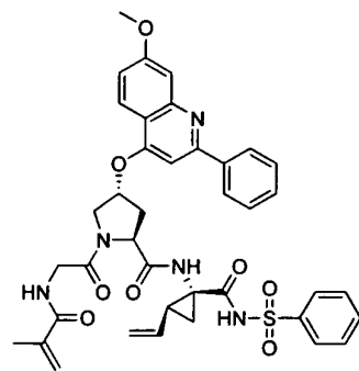
I-44
