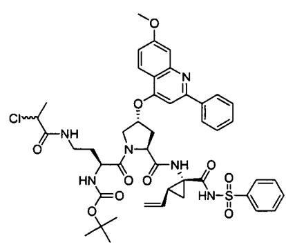
I-1
