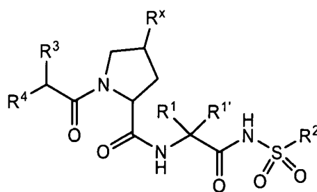
V-b
