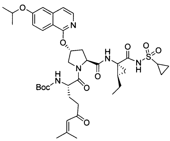
I-117
