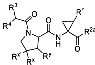
I-d
