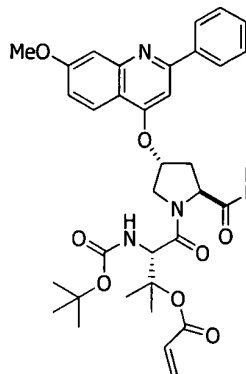
I-40
