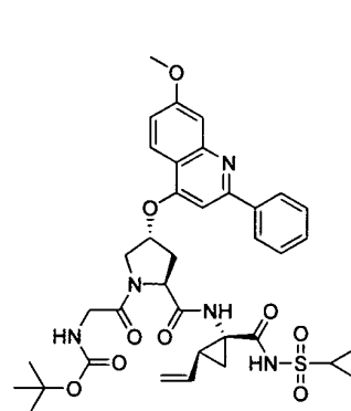
I-38
