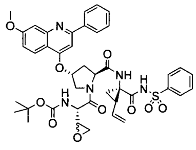
I-14
