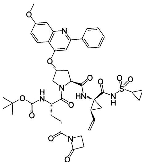
化合物 I-70
