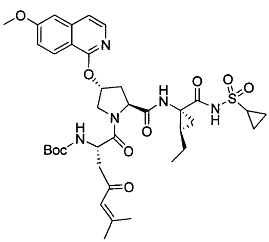
I-119
