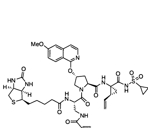
I-103
