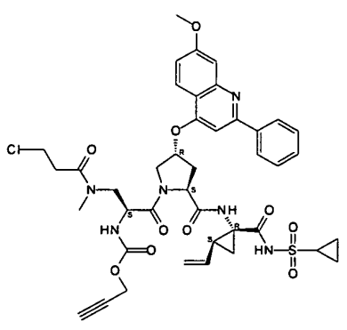
I-71
