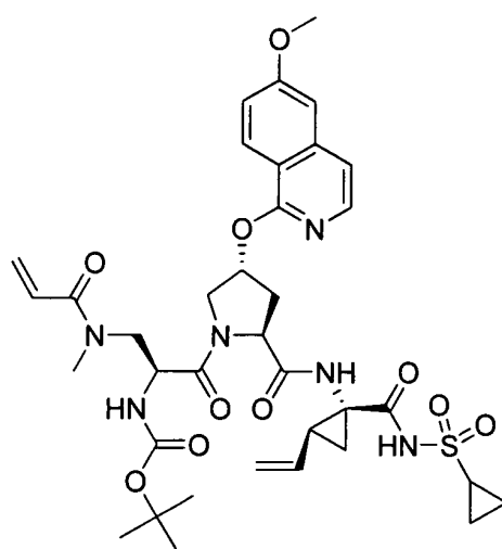
I-93
