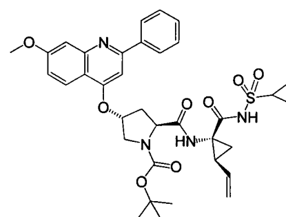
I-62
