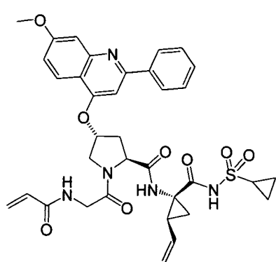
I-39
