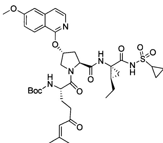
I-114
