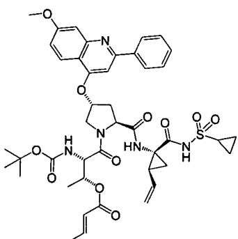
I-50
