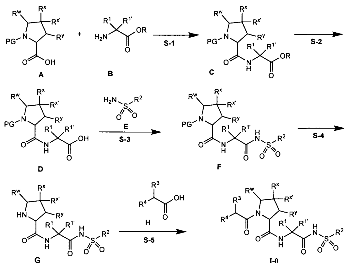
流程 1
