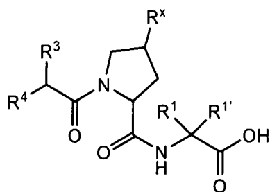
V-a
