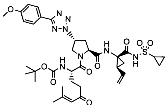
I-107
