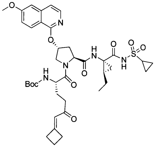
I-122
