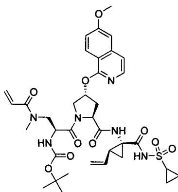
化合物 I-94
