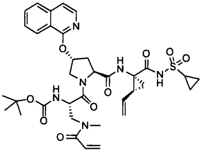
化合物 I-98
