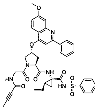
I-43
