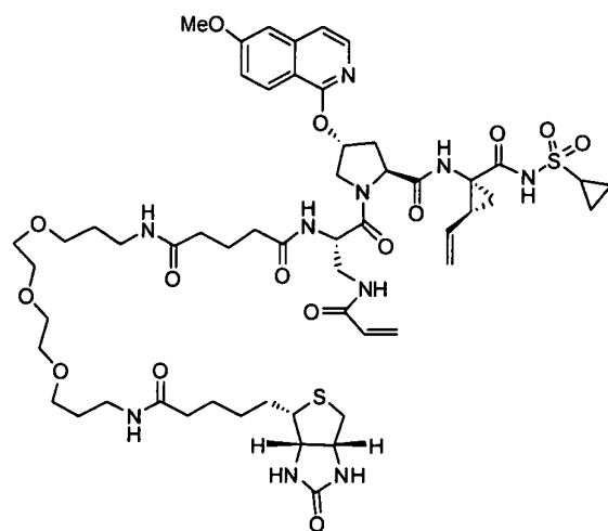
I-104
