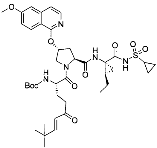
I-123
