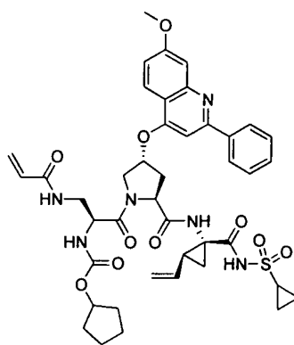
I-55
