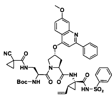
I-11
