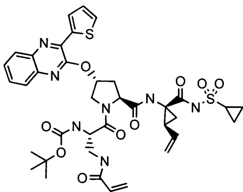
I-109
