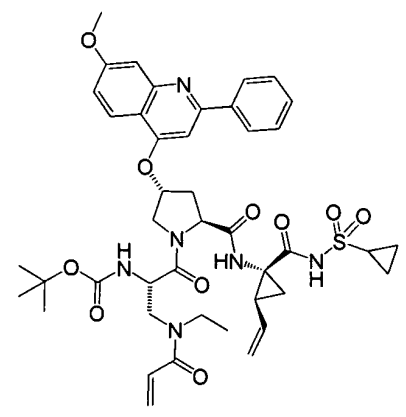
I-78
