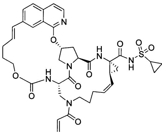
I-111
