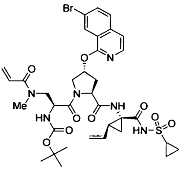
I-84
