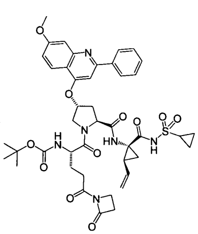
I-70
