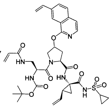
I-76
