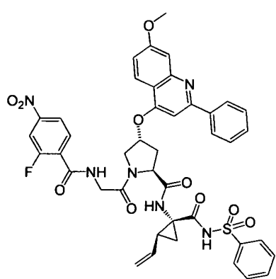
I-63
