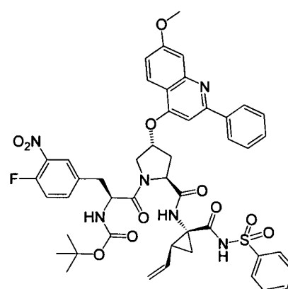
I-59
