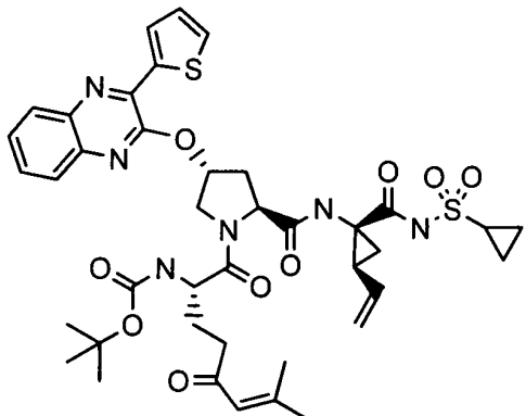
I-110
