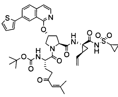
I-87
