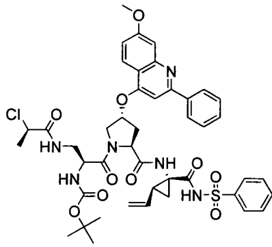
I-13
