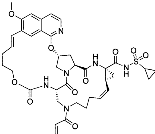
I-113
