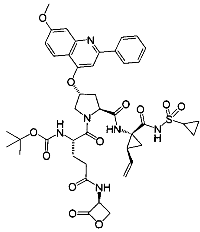
I-69
