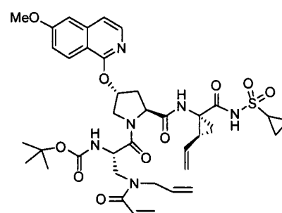
I-99
