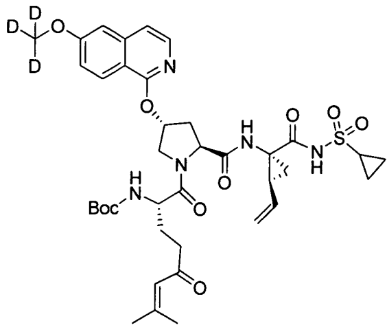
I-116
