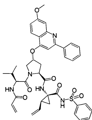
I-60
