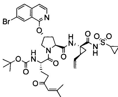
化合物 I-75
