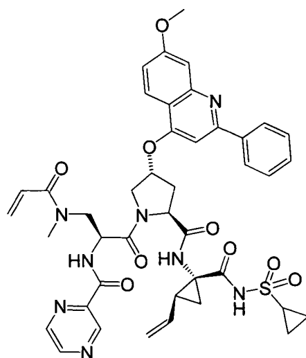
化合物 I-58
