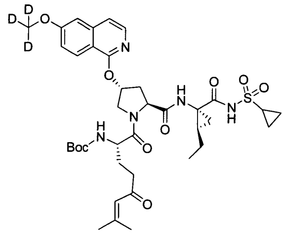
I-118
