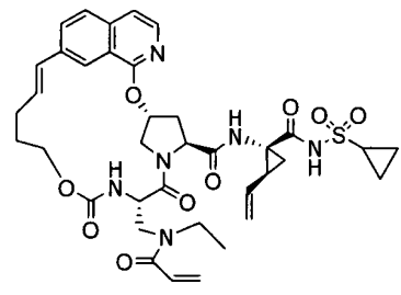
I-15
