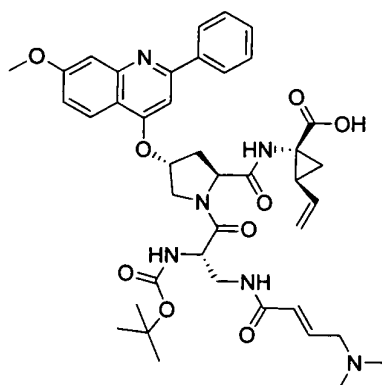
中間體17
