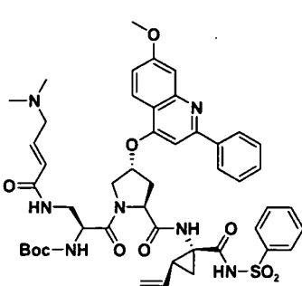
I-5
