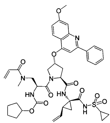
I-72
