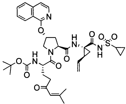
化合物 I-86
