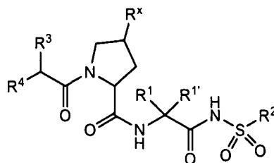
IV-b
