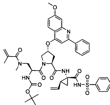
I-32
