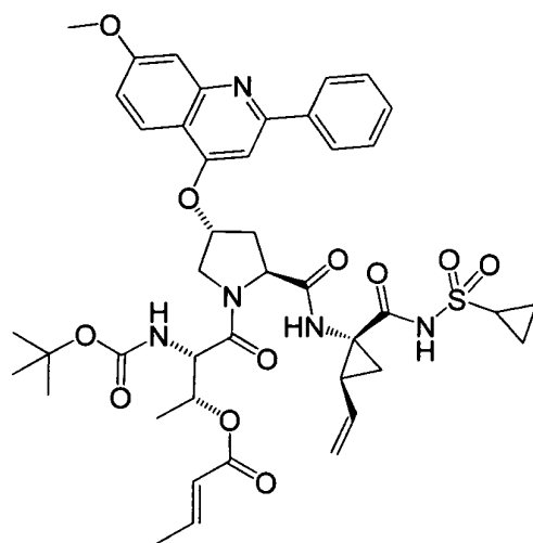
化合物 I-50
