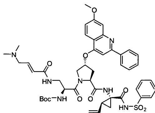
化合物 I-5
