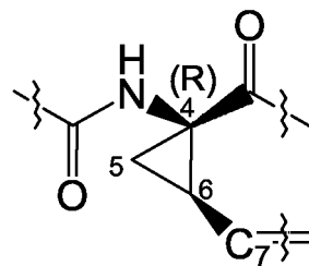
C7 syn to amide
