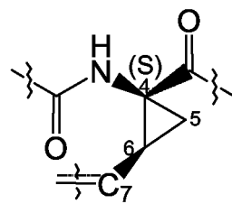
C7 syn to amide
