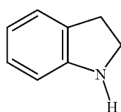
Indoline
