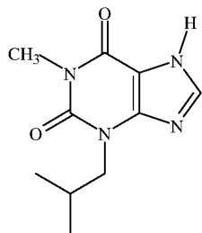
3-isobutyl-1- methylxanthine
