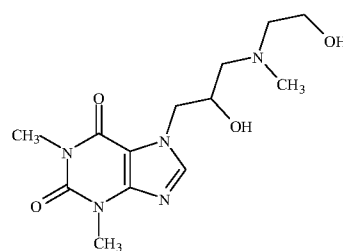
Xanthinol
