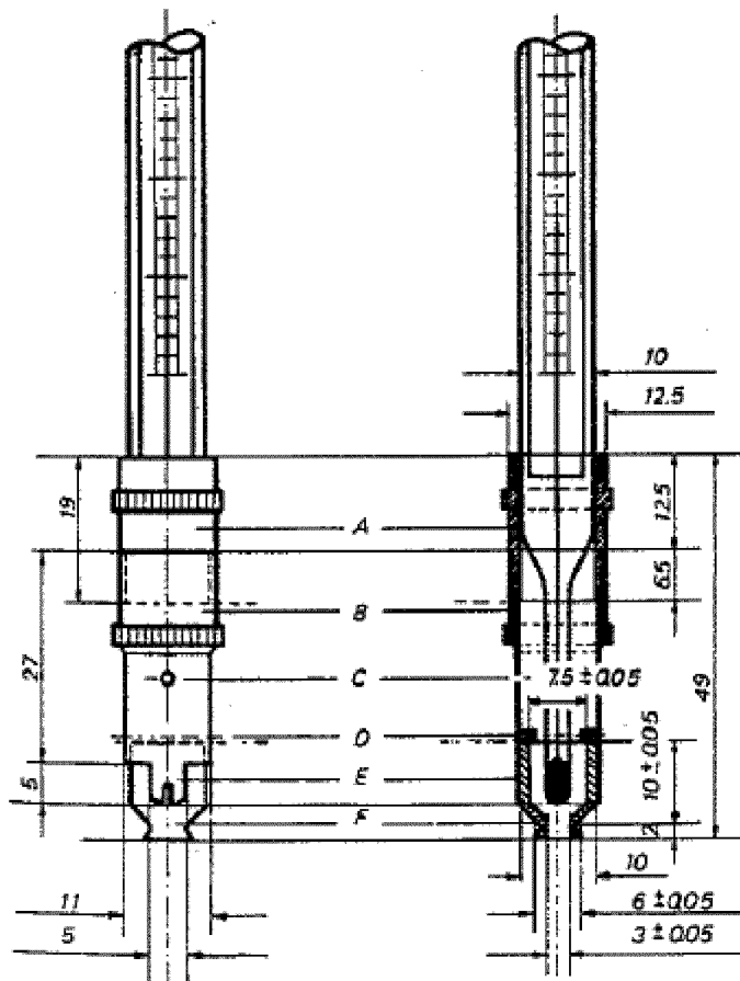
Abb. 2.2.17-1: Apparatur zur Bestimmung des Tropfpunkts Lösungen in Millimetern
