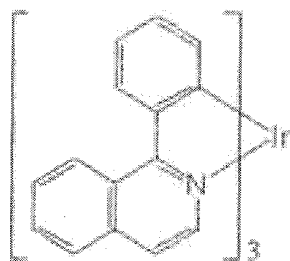
Ir(piq) 3
