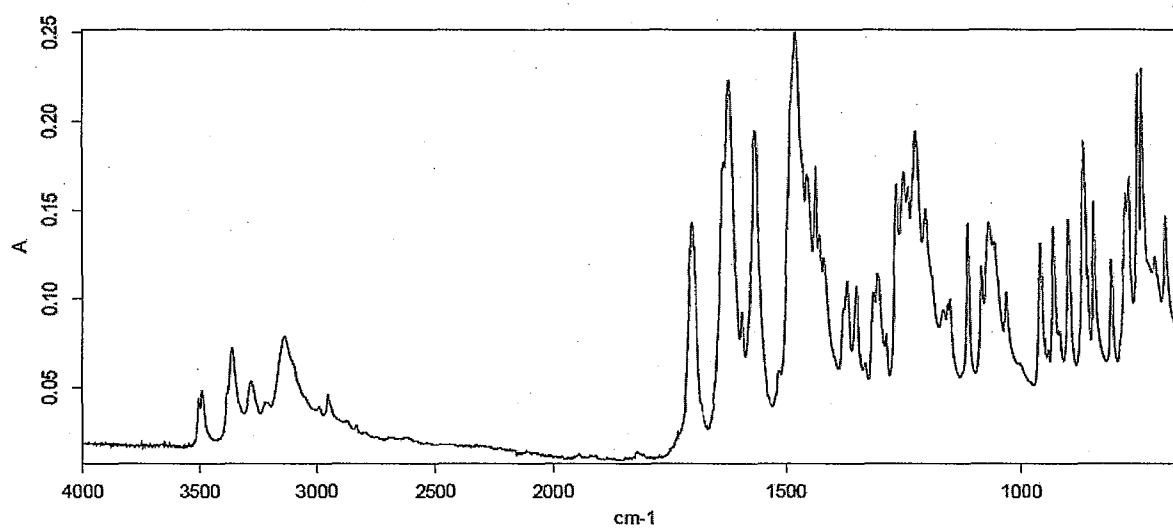
5 Polymorph II
