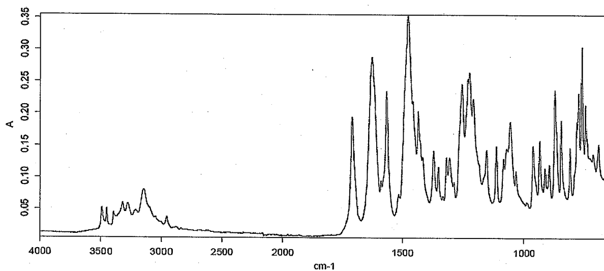
Polymorph V
