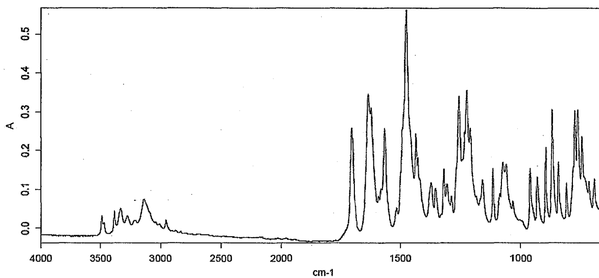
Polymorph I
