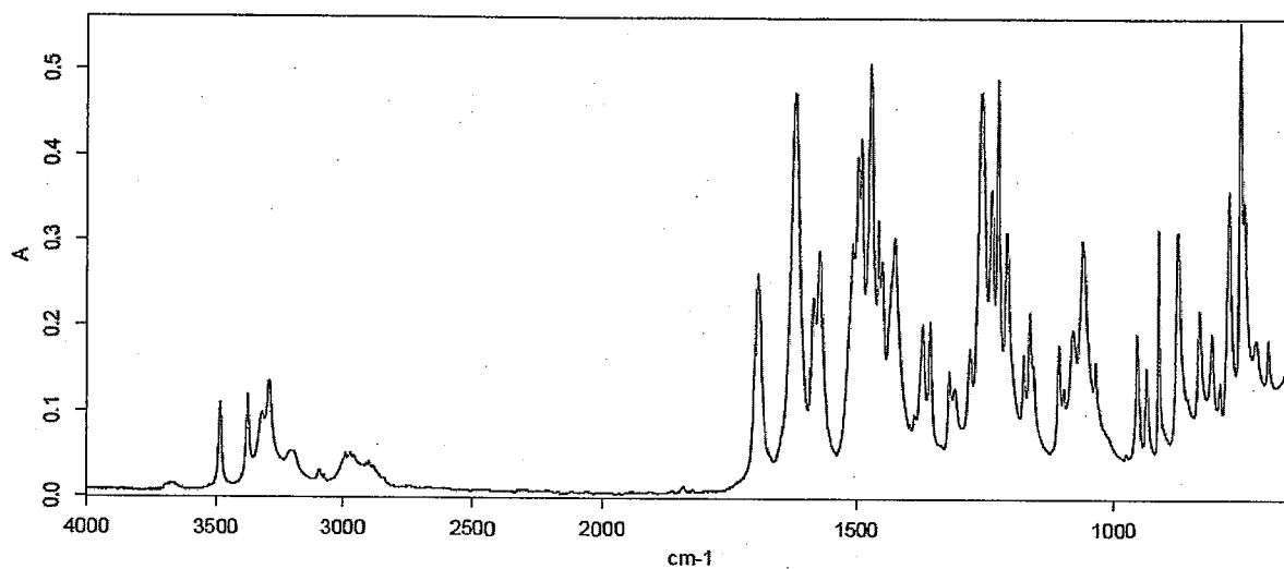
Polymorph IV
