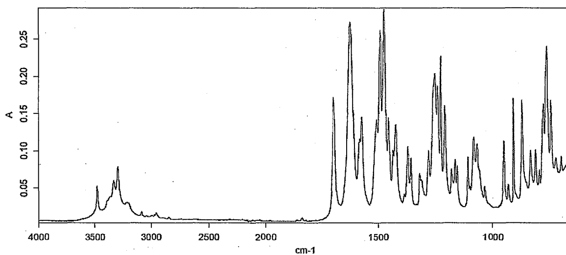
Monohydrate
