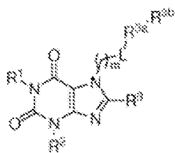
formel VIII
