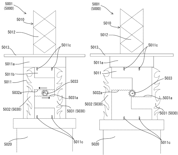
(A) オーラ部材 5030 の閉状態 (B) オーラ部材 5030 の開状態
