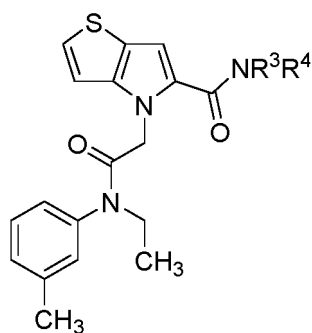
(Ia).
