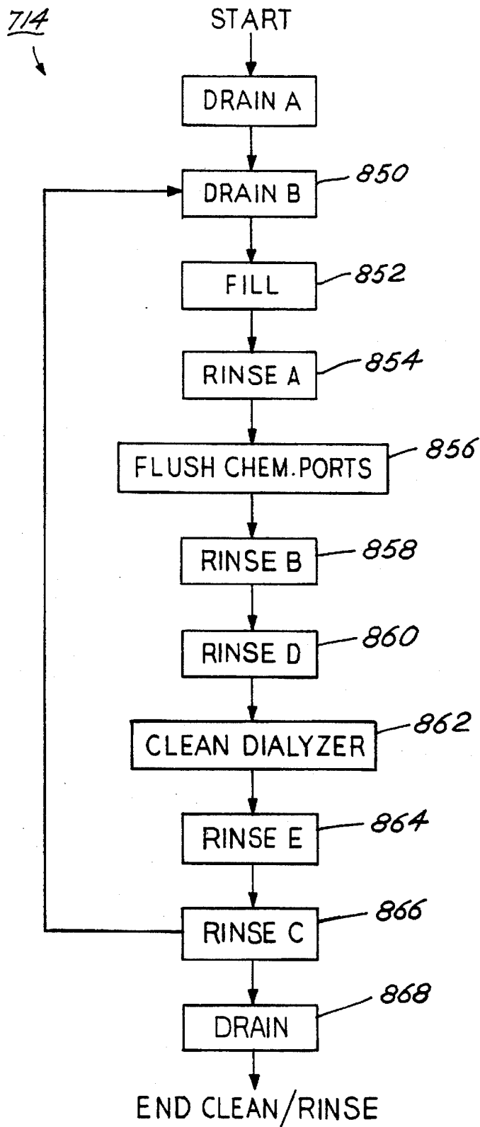
FIG. 23 CLEAN/RINSE
