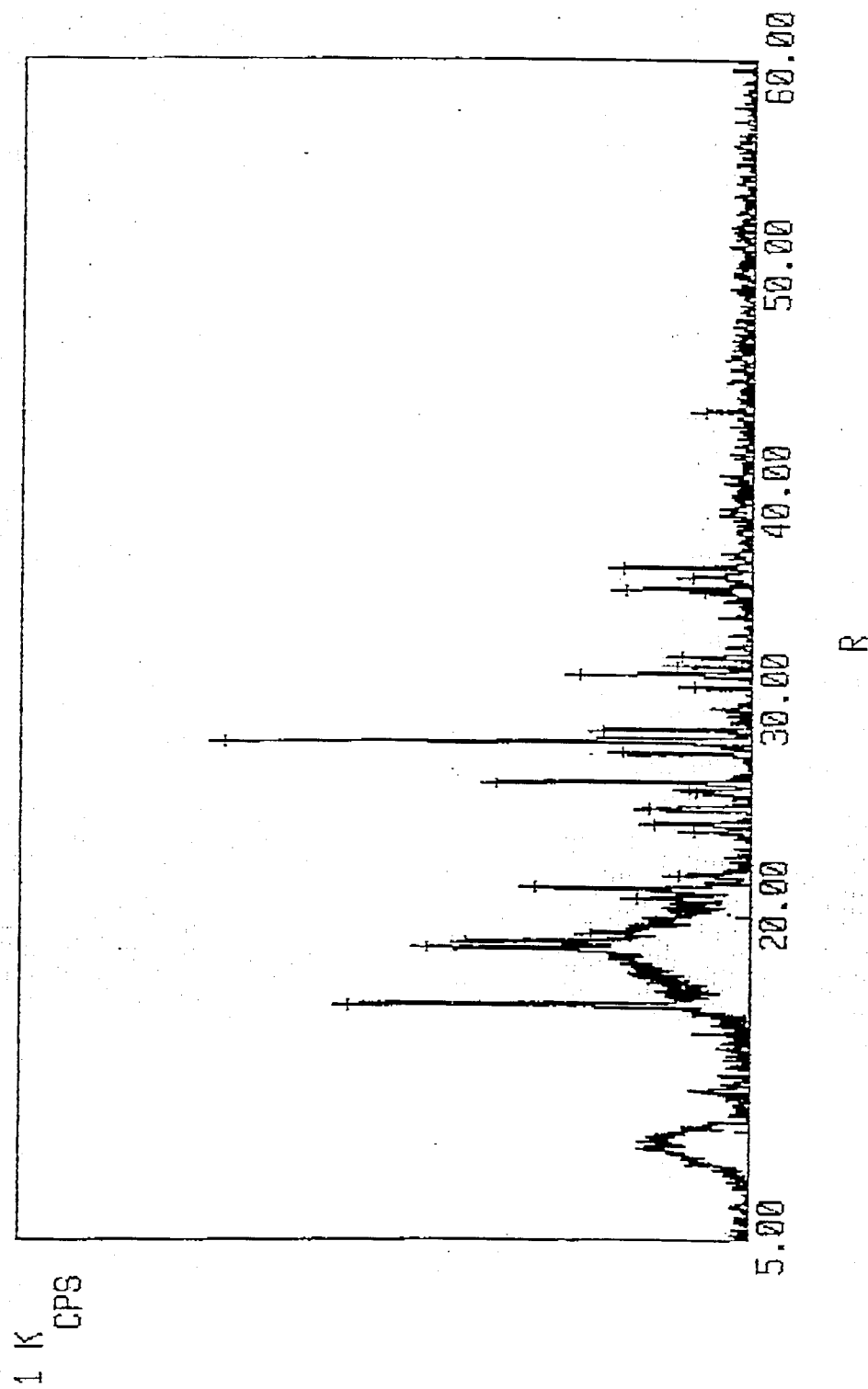
Fig. 3: 5H-MIT.HCl
