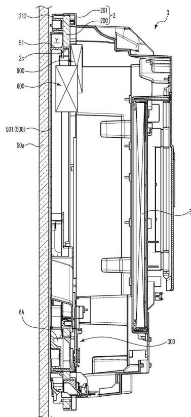
A-A断面図
