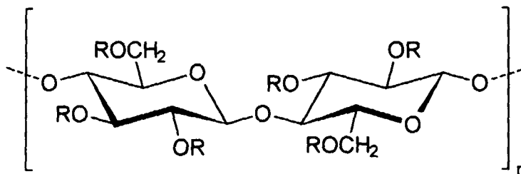
Strukturformel I
