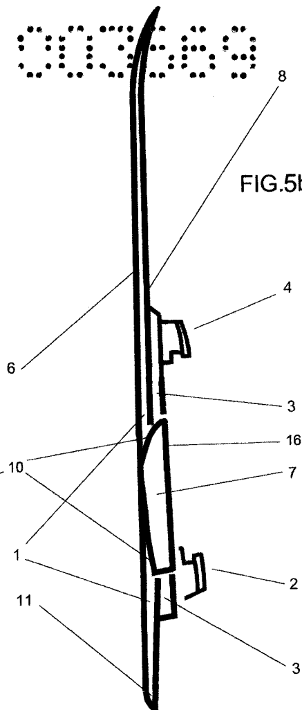
C - C
