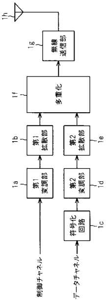
移動機におけるCDMA送信機の構成図
