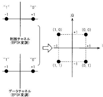
BPSK変調及びIQ複素平面へのマッピング説明図
