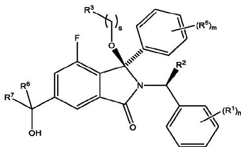
Diastereoisomer 1A
