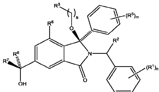
Diastereoisomer 2A
