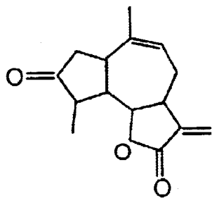
GLABELLIN 17
