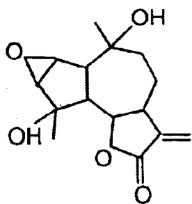
ANOBIN 19
