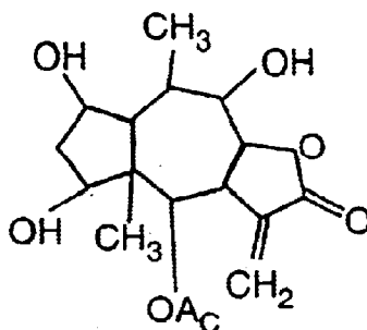
GAIGRANIN 21
