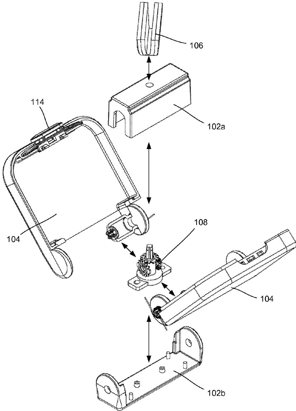
FIG. 1C
