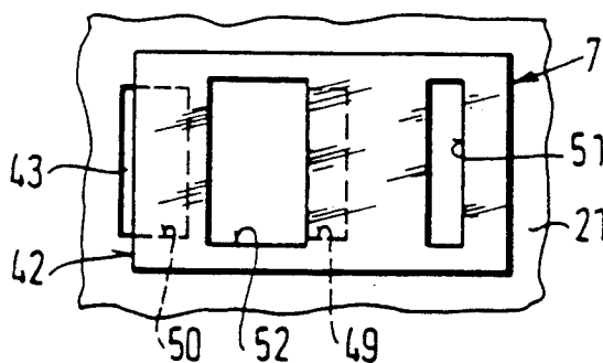
FIG. 7d
