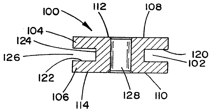
Section A-A FIG. 1c
