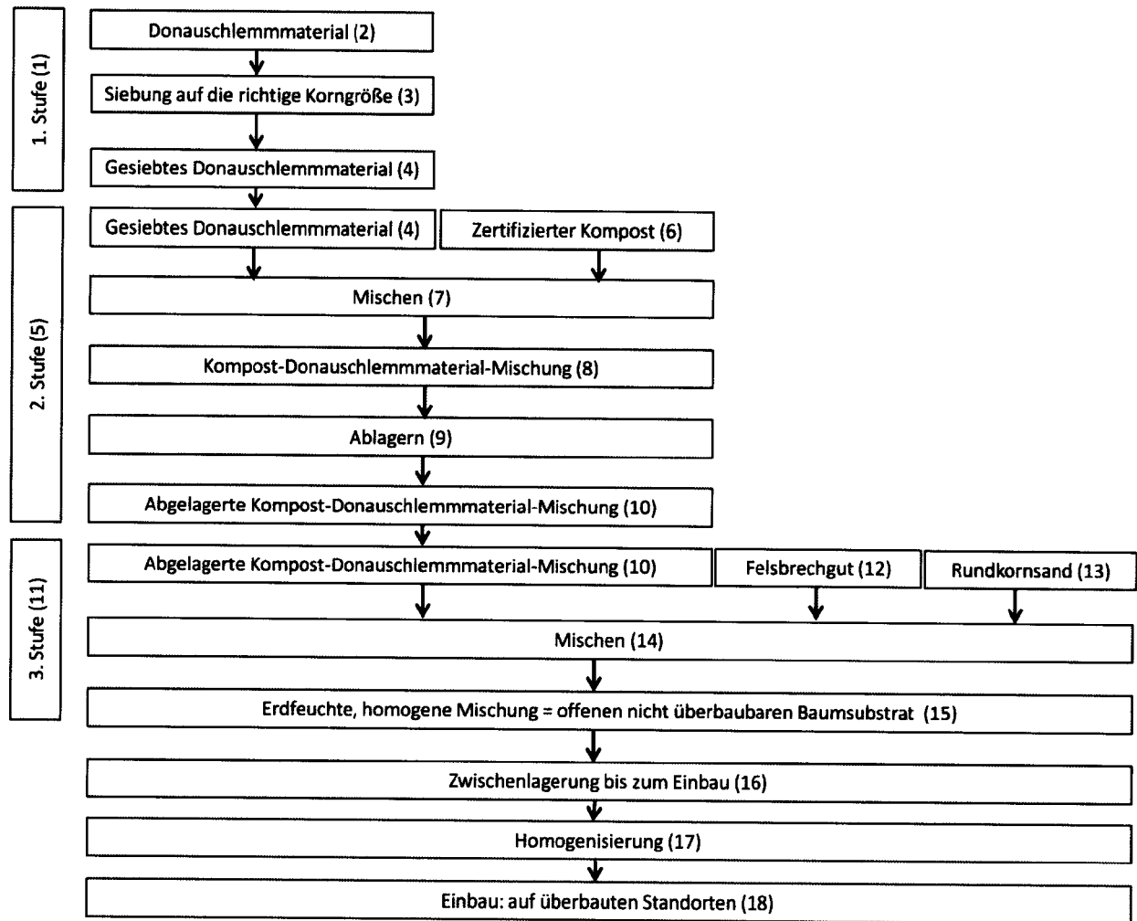
Abb.1: Dreistufiger Misch- und Ablagerungsvorgang (19):
