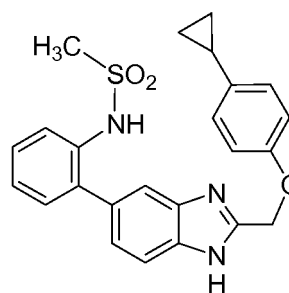
Cpd 168
