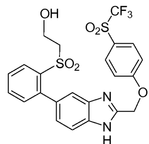
Cpd 161
