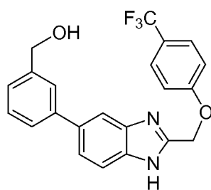
Cpd 117
