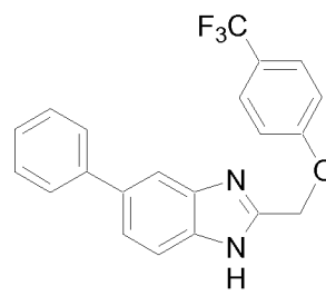
Cpd 126
