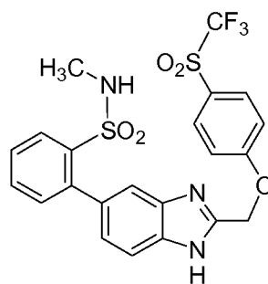
Cpd 20
