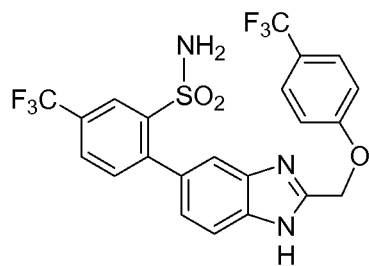
Cpd 133
