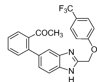
Cpd 49
