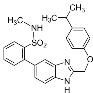
Cpd 51
