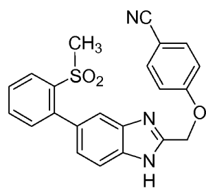
Cpd 83
