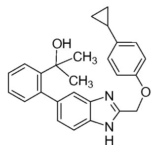
Cpd 163
