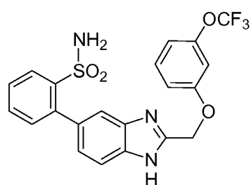
Cpd 15
