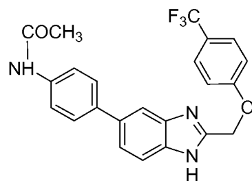
Cpd 115
