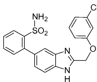
Cpd 6
