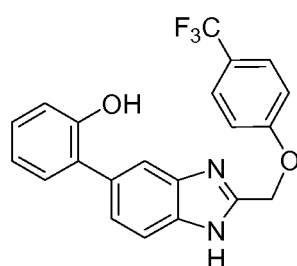
Cpd 119
