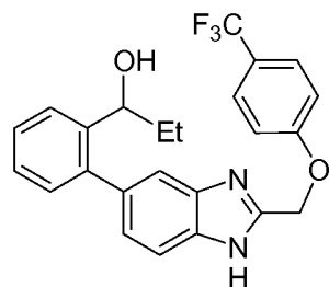
Cpd 143
