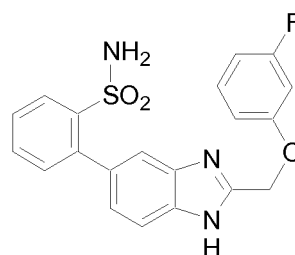
Cpd 4
