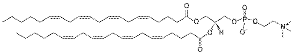
(DAPC);
