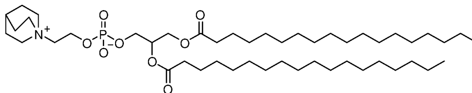
Cmpd H 420
