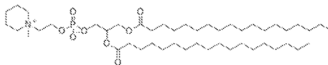
Cmpd H 419
