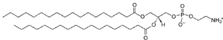
(DSPE);
