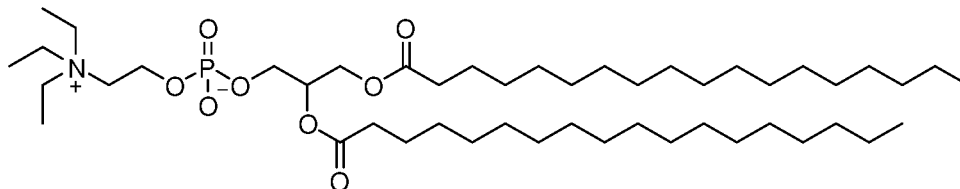
DMPC
