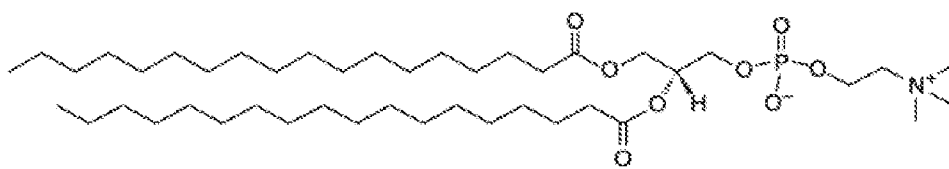
(DSPC);
