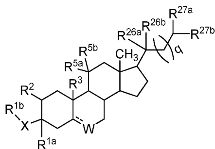
Formula SVII,
