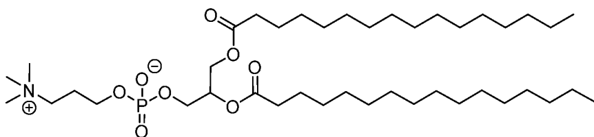
(Cmpd H 154)
