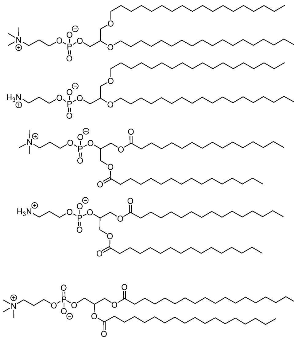
(Cmpd H 162)
