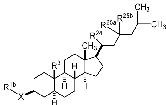
Formula SVIb,
