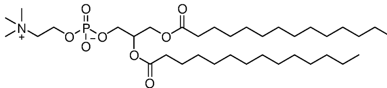
DPPC
