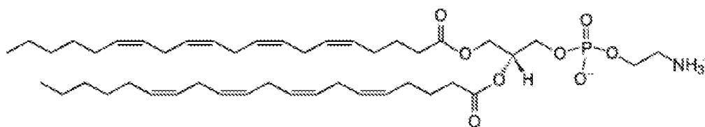
DAPE;
