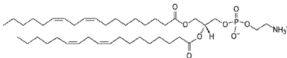
PE 18:2/18:2;
