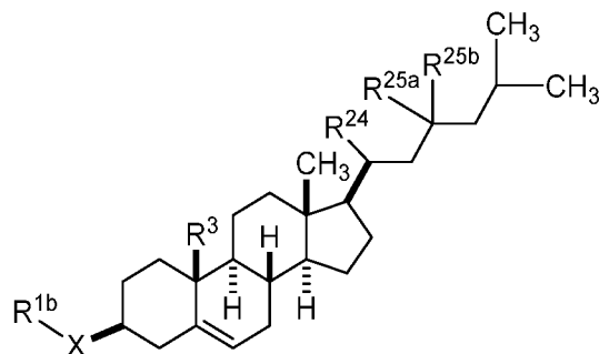
Formula SVIa,
