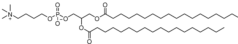
Cmpd H 420
