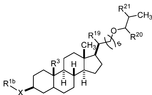
Formula SIVb,
