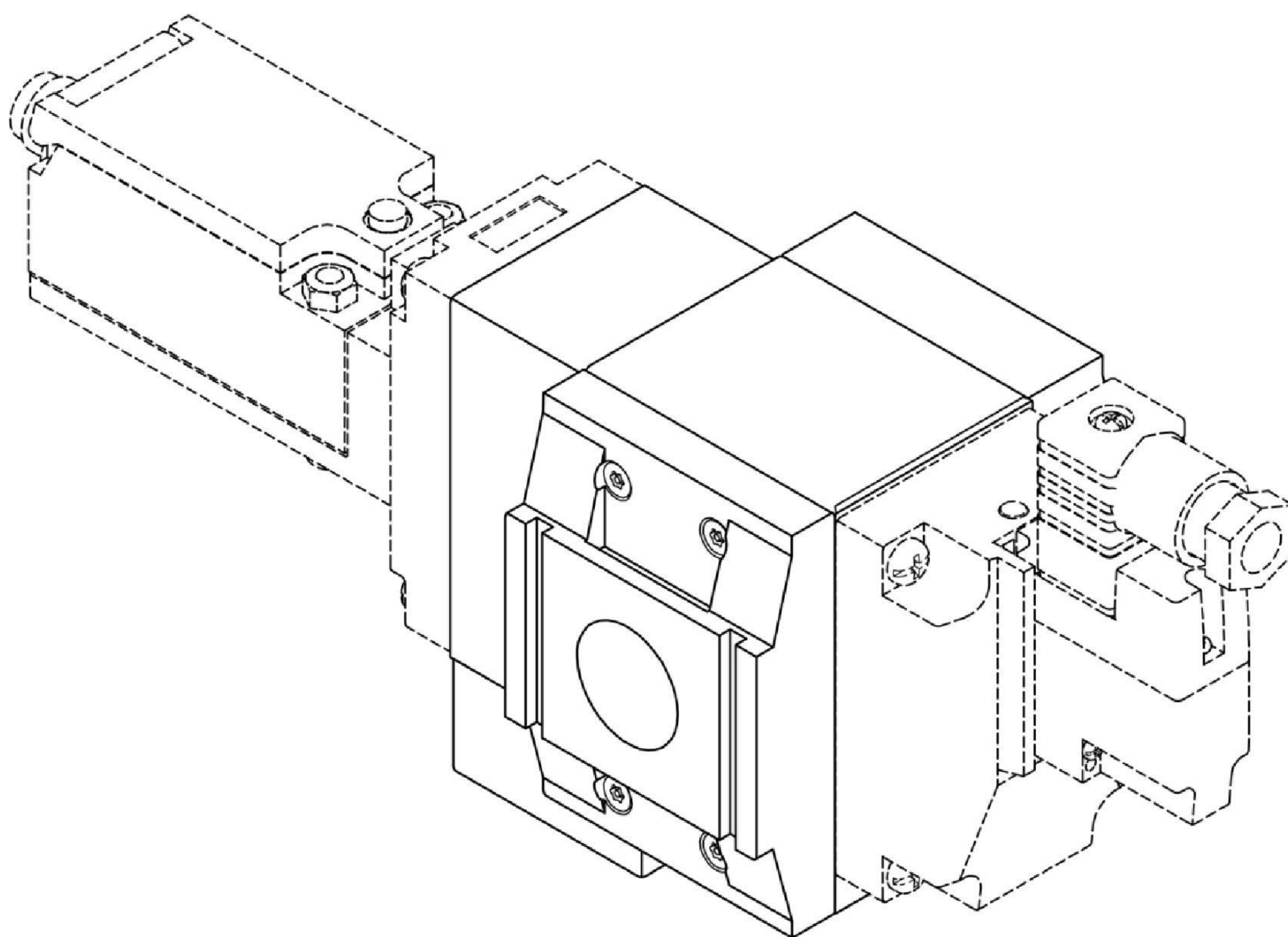
【立體圖 1】
