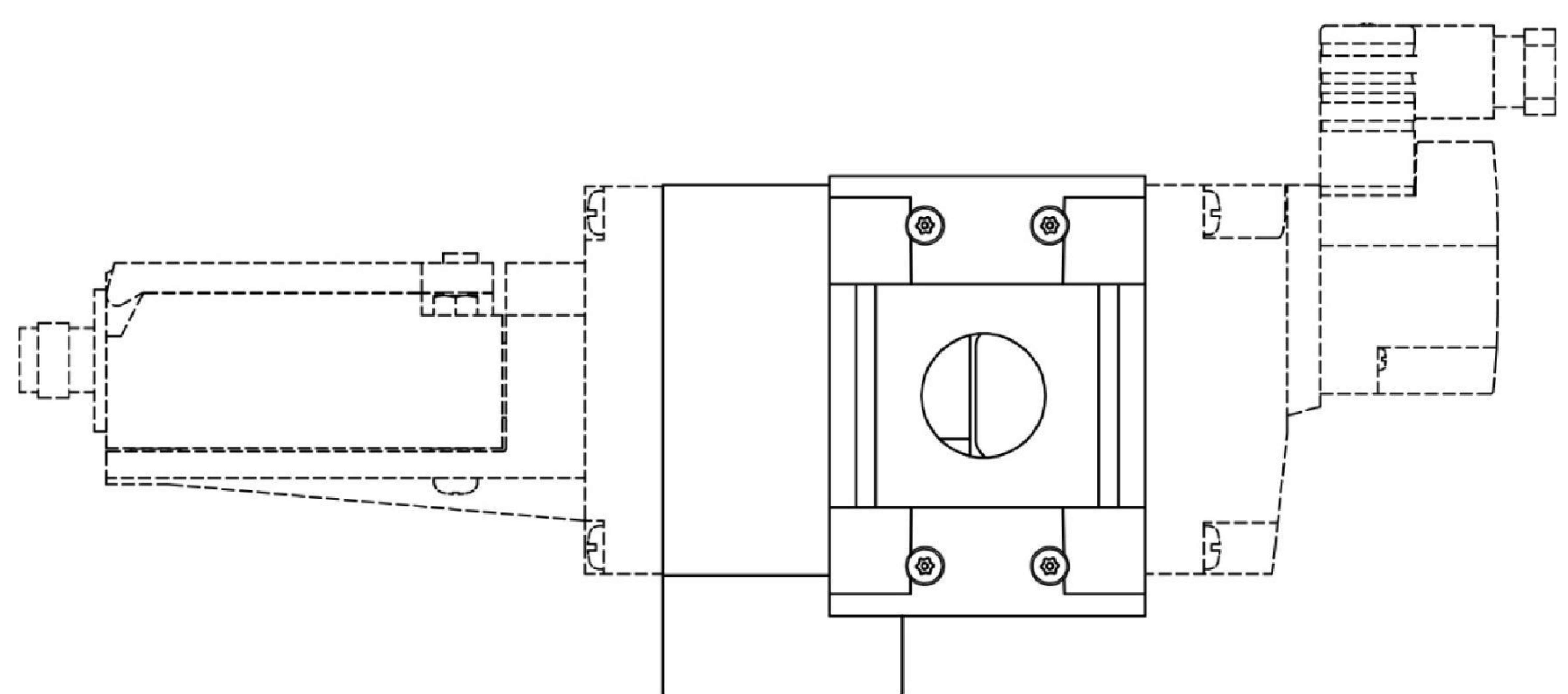
【後視圖】
