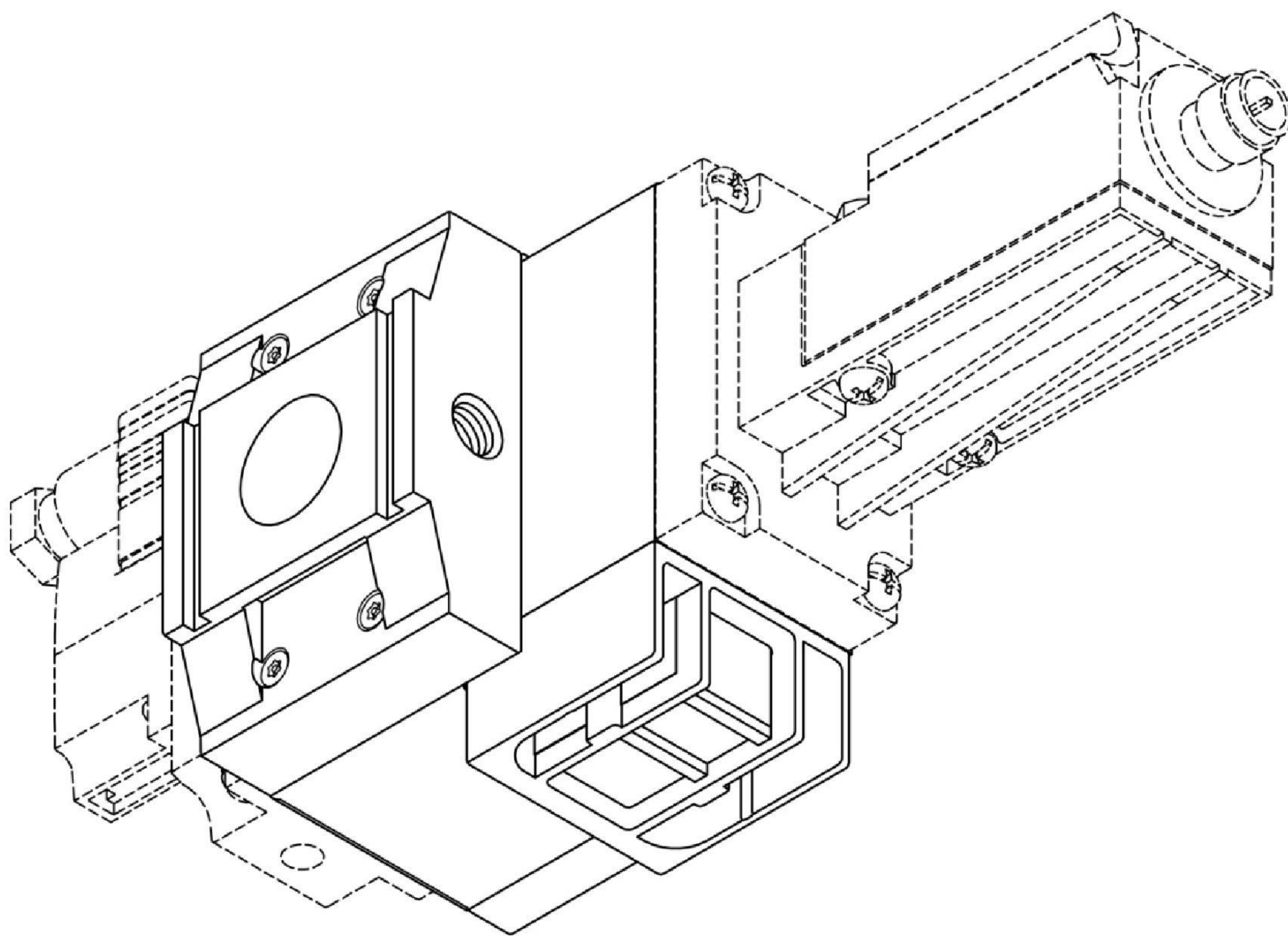
【立體圖 2】
