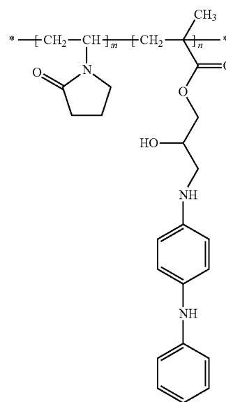
P(VP-ANi)
