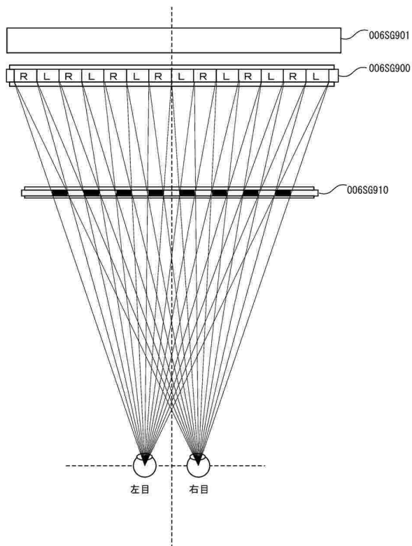
【図13-44】 変形例006SG-7
