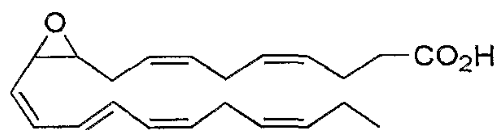
10,11-Epoxy-DHA
