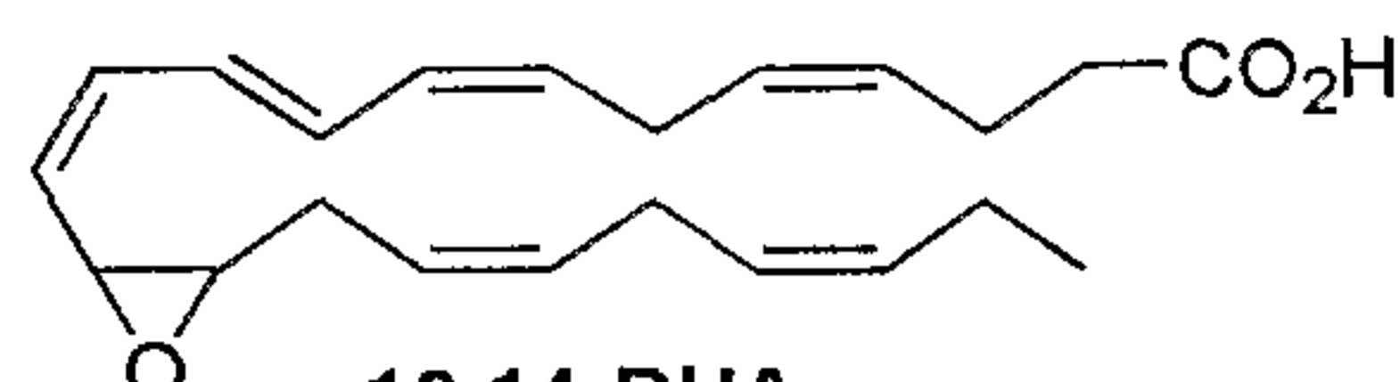
13,14-DHA
