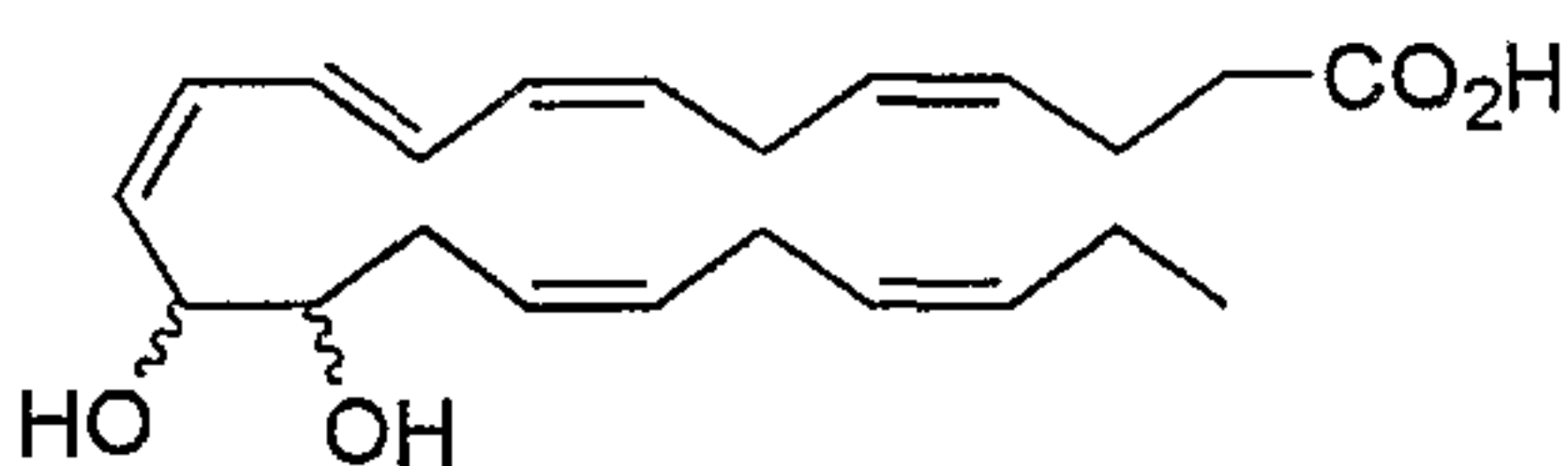
13,14-DihydroxyDHA
