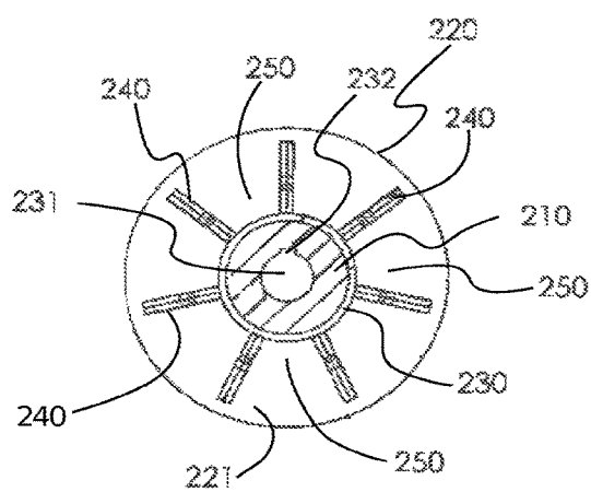
FIG. 3 A-A
