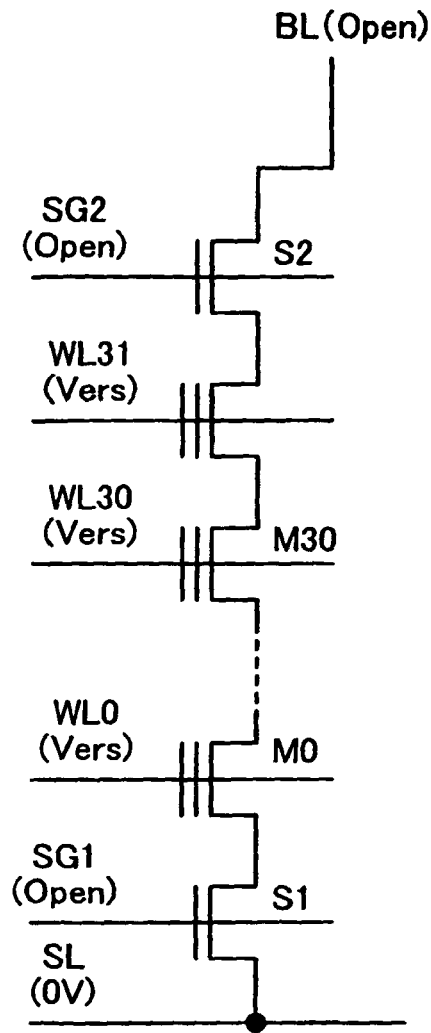
FIG. 20A erasing
