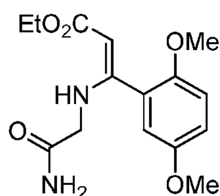
(Z)-Ethyl 3-((2-amino-2-oxoethyl)amino)-3-(2,5-dimethoxyphenyl)acrylate
