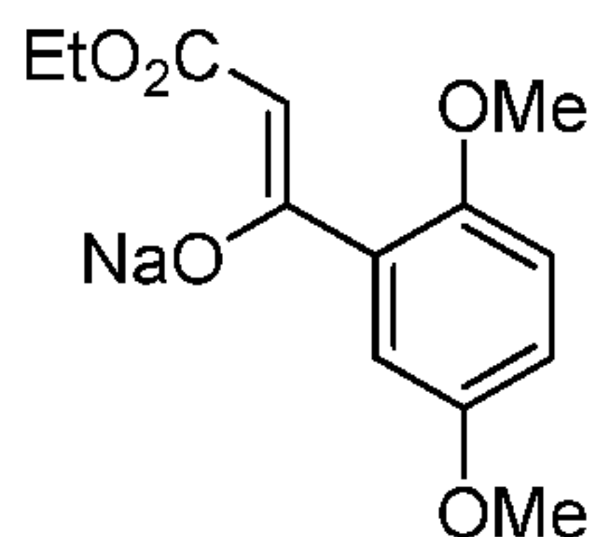
Sodium 1-(2,5-dimethoxyphenyl)-3-ethoxy-3-oxoprop-1-en-1-olate
