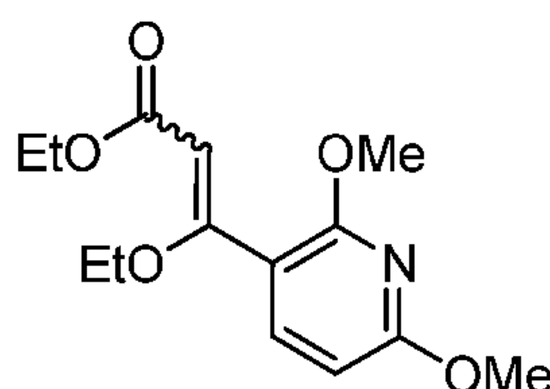
(Z,E)-Ethyl 3-(2,6-dimethoxypyridin-3-yl)-3-ethoxyacrylate
