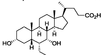
обетихолевая кислота (ХА)
