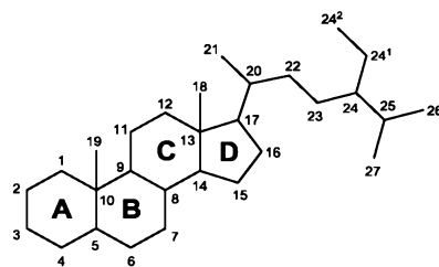
общая система нумерации стероидов
