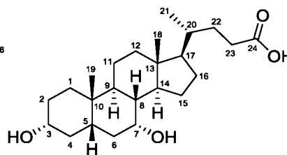
Нумерация в ХДХК
