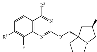
Formula II-2-A
