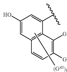
F-3-B
