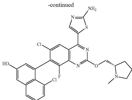
121
