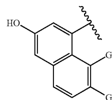
F-3-A
