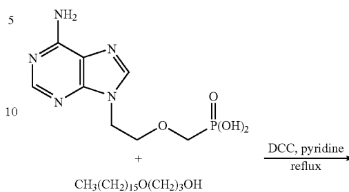
Scheme VI
