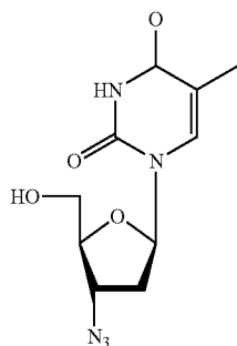
AZT
