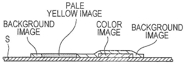
FIG. 9B
